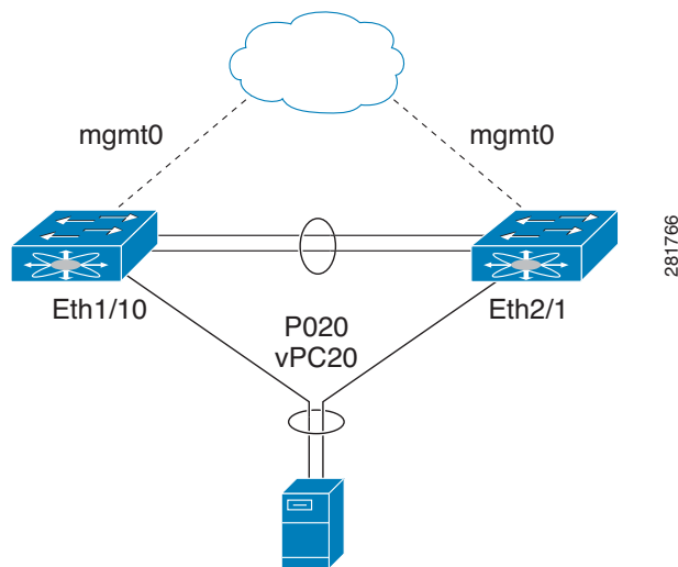
図 1-4 スイッチ vPC トポロジ
