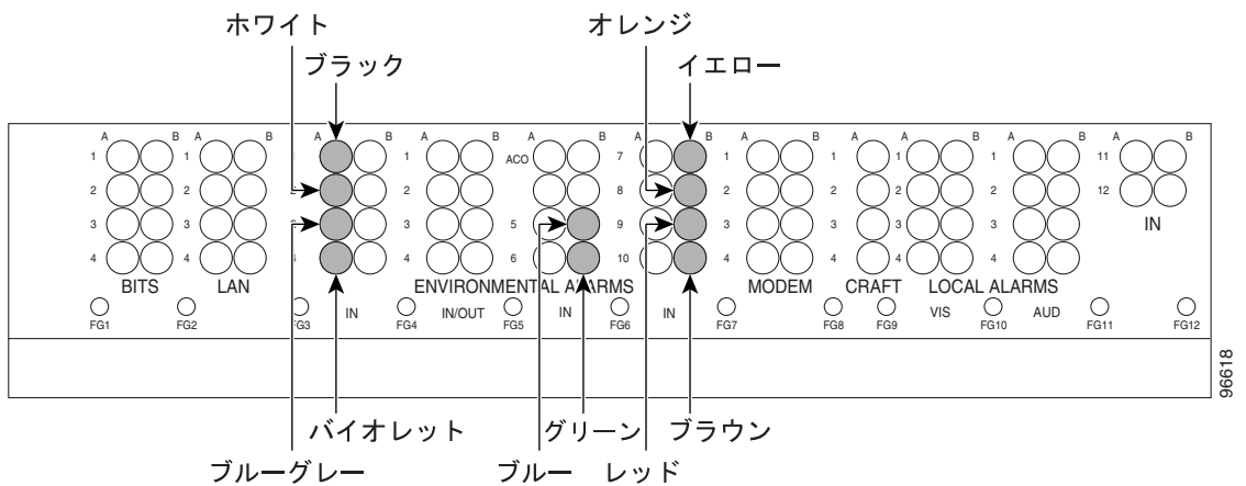
図 1-30 バックプレーンピンへの AEP ワイヤラップ接続
