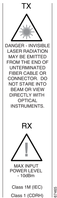
図 4-16 OC192 LR/STM64 LH 1550 (15454-OC192LR1550) 前面プレートの拡大図
