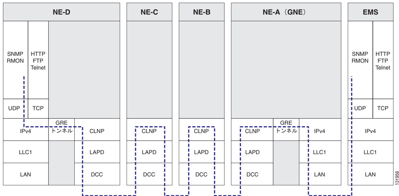
図 13-27 IP-over-CLNS トンネル フロー
