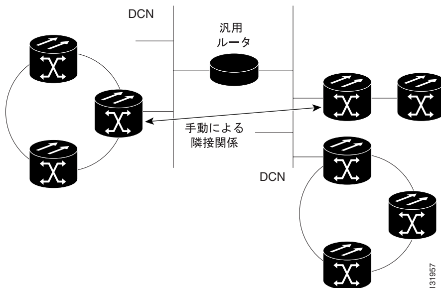
図 13-23 手動による TARP 隣接関係
