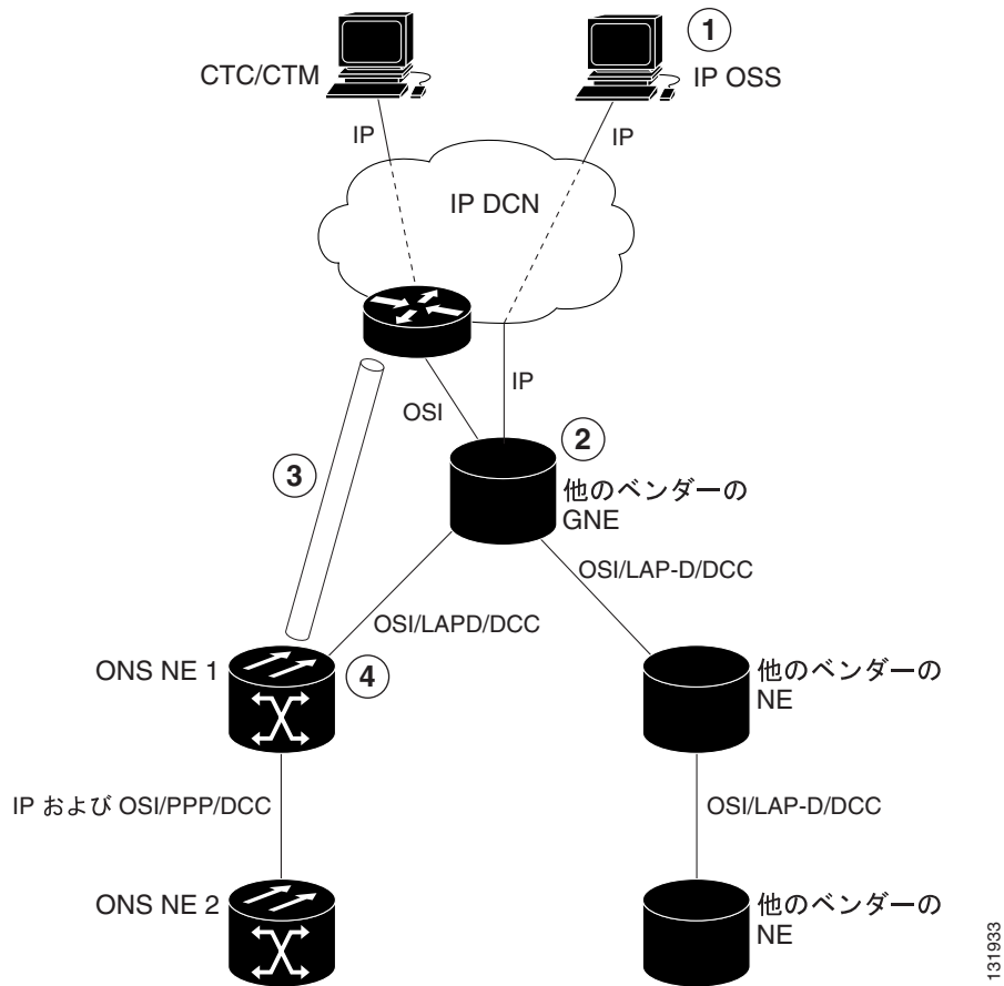
図 13-33 OSI/IP のシナリオ 3 : IP OSS、IP DCN、他のベンダーの GNE、OSI DCC、および ONS ENE
