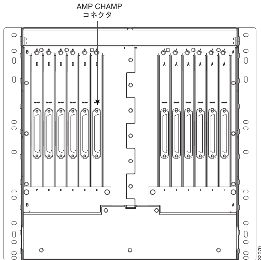
図 1-19 AMP Champ EIA のバックプレーン
