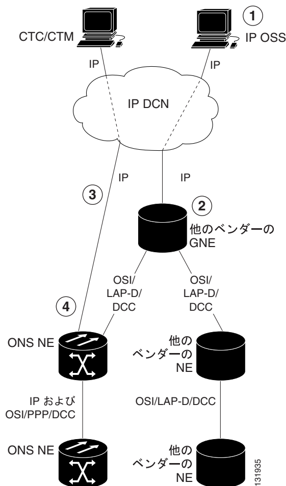
図 13-36 OSI/IP のシナリオ 5 : OSI DCC 接続を使用しない GNE
