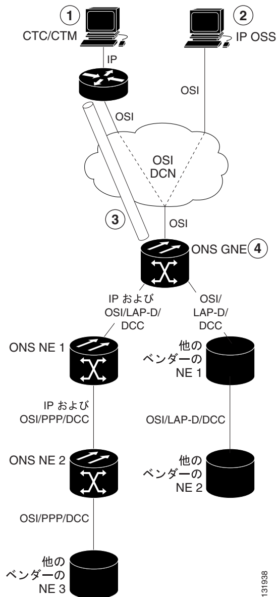
図 13-39 OSI/IP のシナリオ 8 : OSI OSS、OSI DCN、ONS GNE、OSI DCC、および他のベンダーの NE
