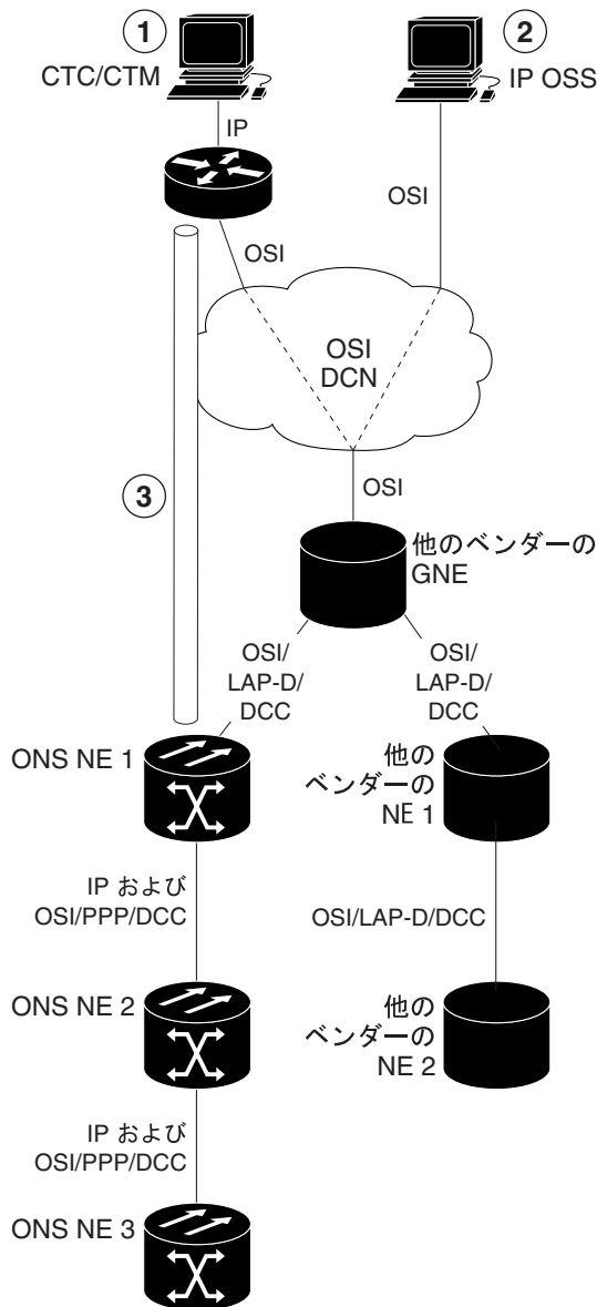
図 13-38 OSI/IP のシナリオ 7: OSI OSS、OSI DCN、他のベンダーの GNE、OSI DCC、および ONS NE
