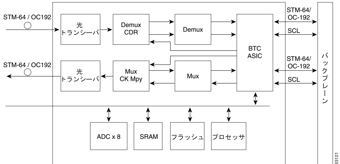
図 4-20 OC192 LR/STM64 LH ITU 15xx.xx カードのブロック図
