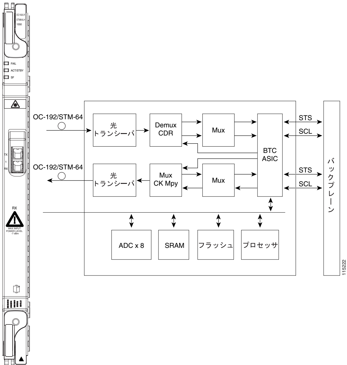
図 4-17 OC192 LR/STM64 LH 1550 ( 15454-OC192-LR2 ) カードの前面プレートとブロック図
