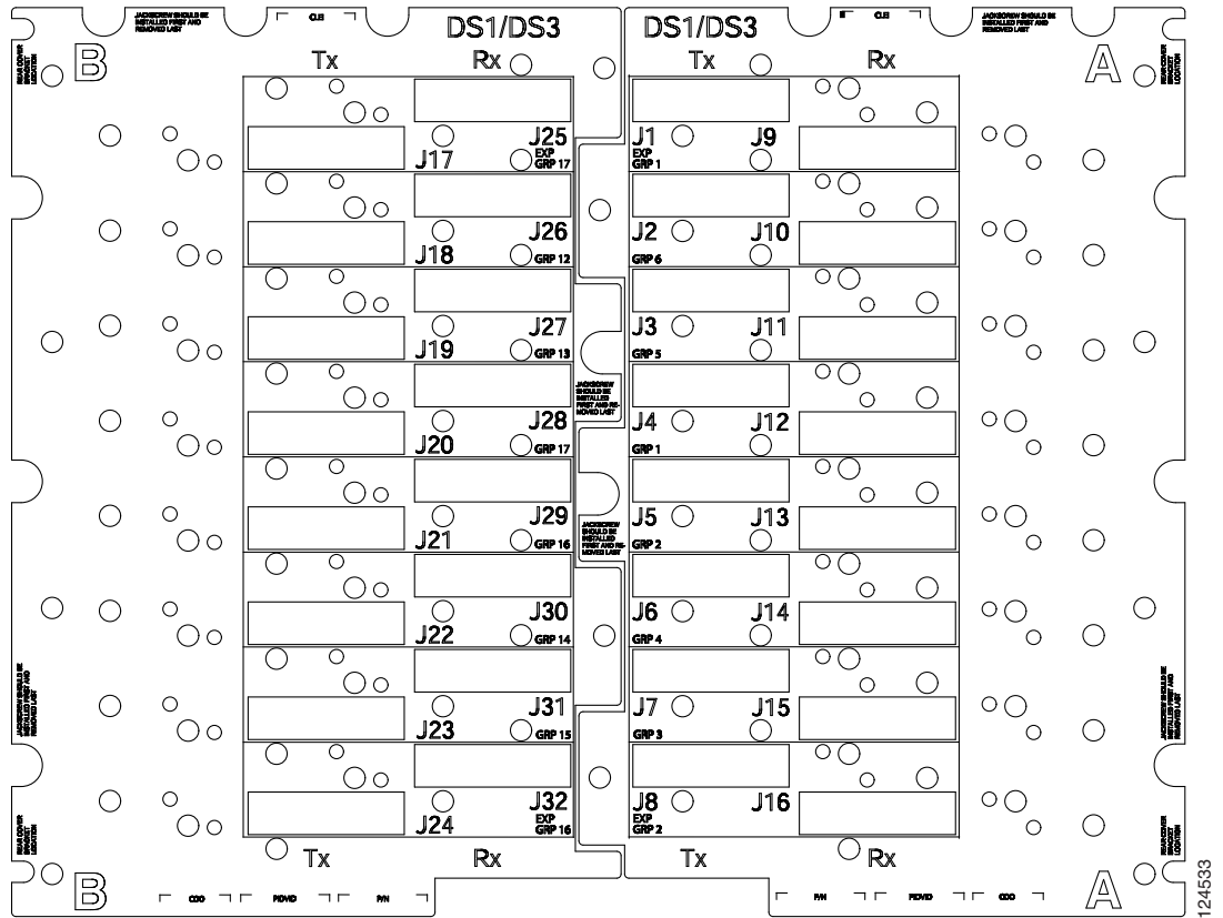
図 1-21 UBIC-H EIA のコネクタ ラベル
