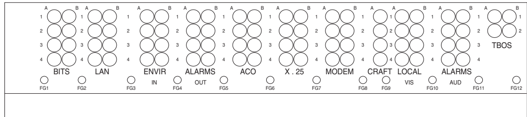
図 1-36 ONS 15454 バックプレーンのピン割り当て
