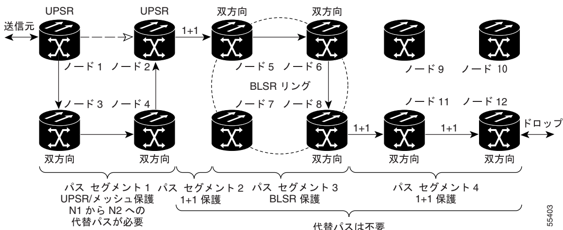
図 11-10 仮想 UPSR セグメントの代替パス
