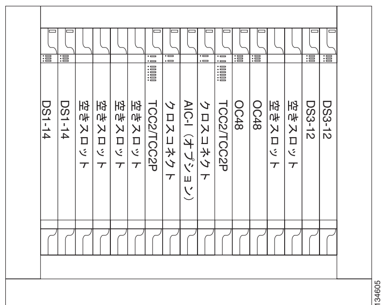
図 12-10 図 12-8 のノード 1 ~ 4 のシェルフ アセンブリ レイアウト
