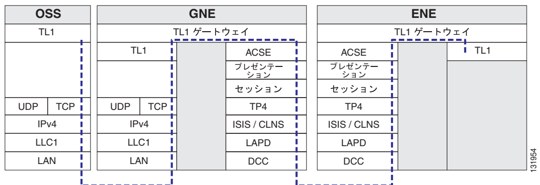
図 13-24 T-TD プロトコルフロー
