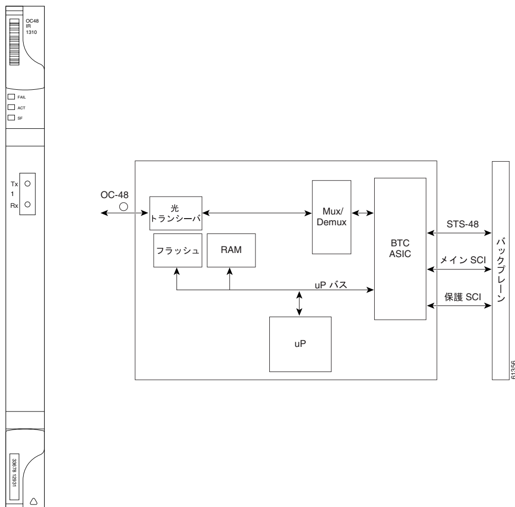
図 4-7 OC48 IR 1310 カードの前面プレートとブロック図
