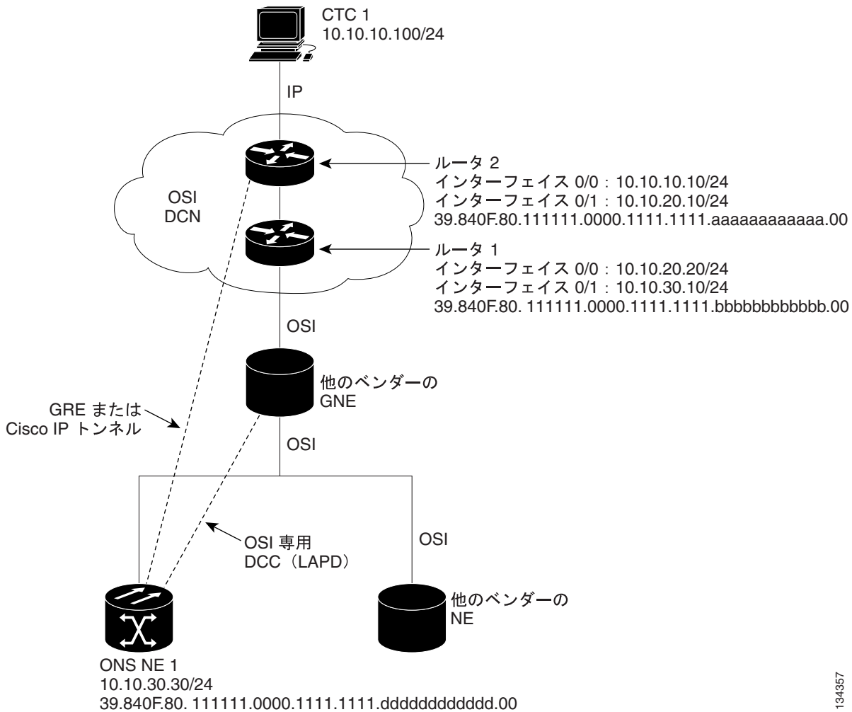
図 13-30 IP-over-CLNS トンネルのシナリオ 3 : ONS ノードから OSI DCN 上のルータへ
