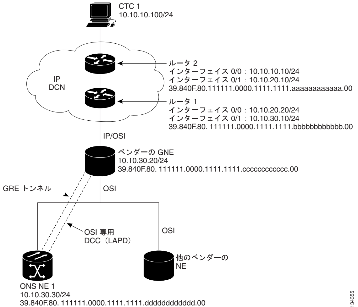
図 13-28 IP-over-CLNS トンネルのシナリオ 1 : ONS NE から他のベンダーの GNE へ
