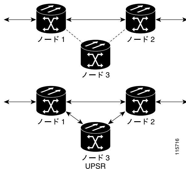
図 12-32 非保護のポイントツーポイントまたはリニア ADM から UPSR への変換
