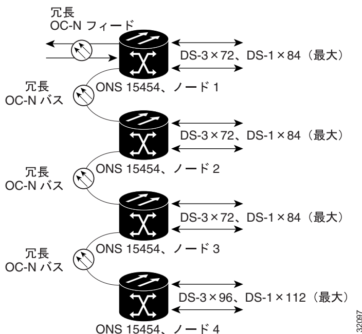
図 12-31 4 シェルフ ノード構成
