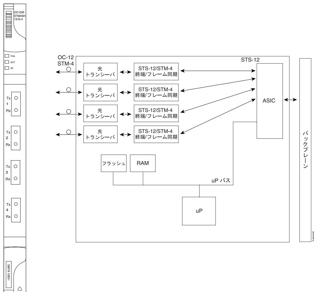
図 4-6 OC12 IR/STM4 SH 1310-4 カードの前面プレートとブロック図
