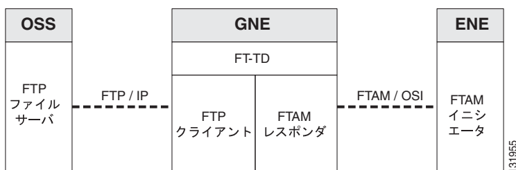
図 13-25 FT-TD プロトコルフロー
