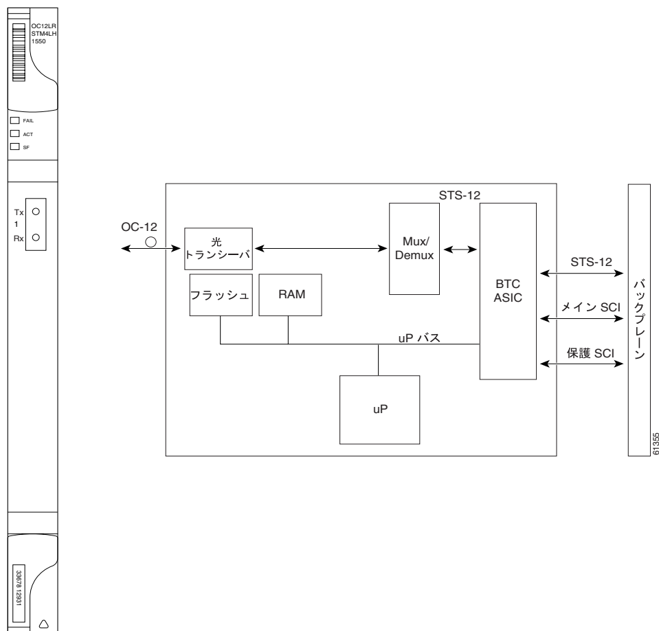
図 4-5 OC12 LR/STM4 LH 1550 カードの前面プレートとブロック図
