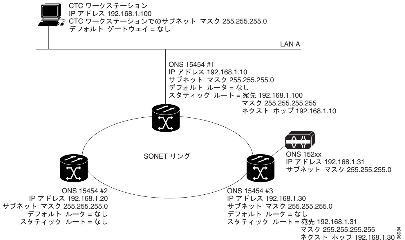
図 13-4 IP のシナリオ 3 : スタティックルーティングでのプロキシ ARP の使用
