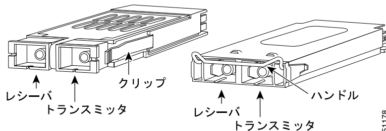
図 5-10 クリップ付き (左) とハンドル付き (右) の GBIC
