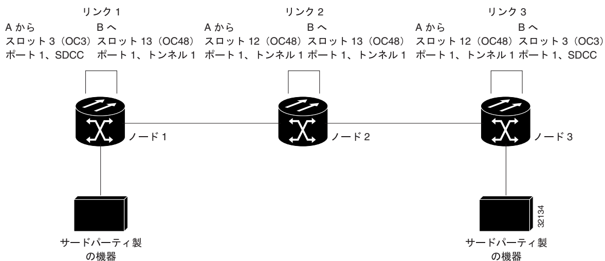
図 11-5 従来の DCC トンネル
