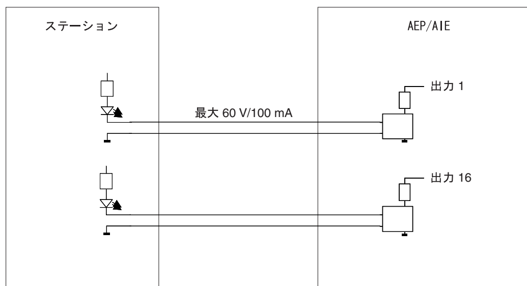
図 1-32 アラーム出力の回路図
