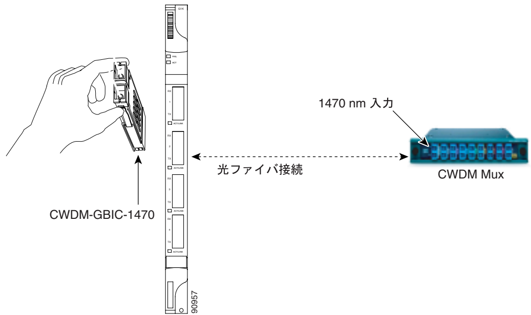
図 5-11 光接続装置に適した波長の CWDM GBIC
