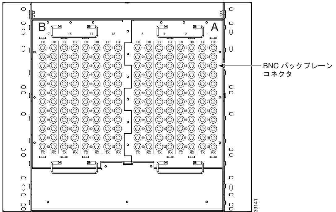
図 1-15 1:N 保護スキームで使用する高密度 BNC バックプレーン
