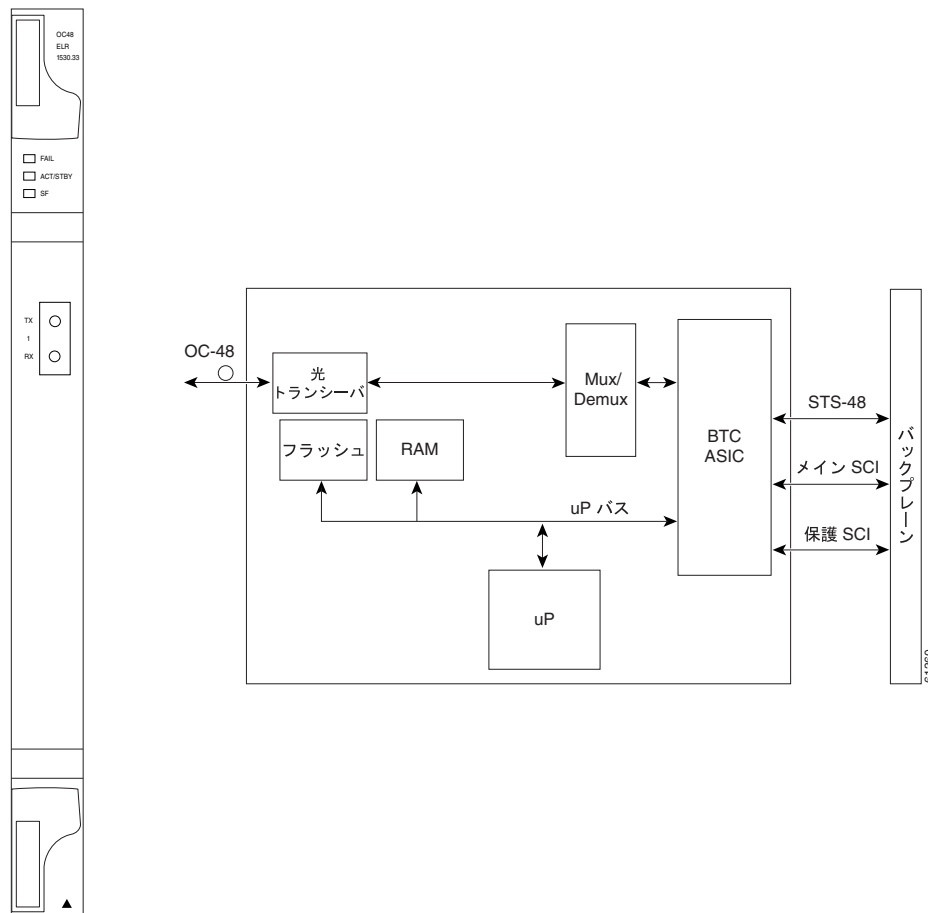
図 4-12 OC48 ELR 200 GHz カードの前面プレートとブロック図
