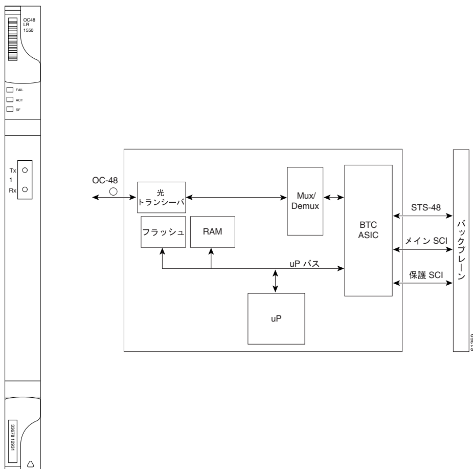
図 4-8 OC48 LR 1550 カードの前面プレートとブロック図
