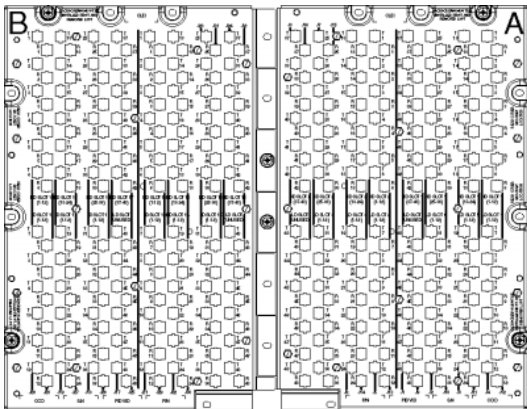
図 1-16 1:N 保護スキームで使用する MiniBNC バックプレーン
