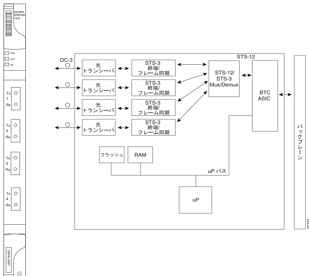
図 4-1 OC3 IR 4/STM1 SH 1310 カードの前面プレートとブロック図
