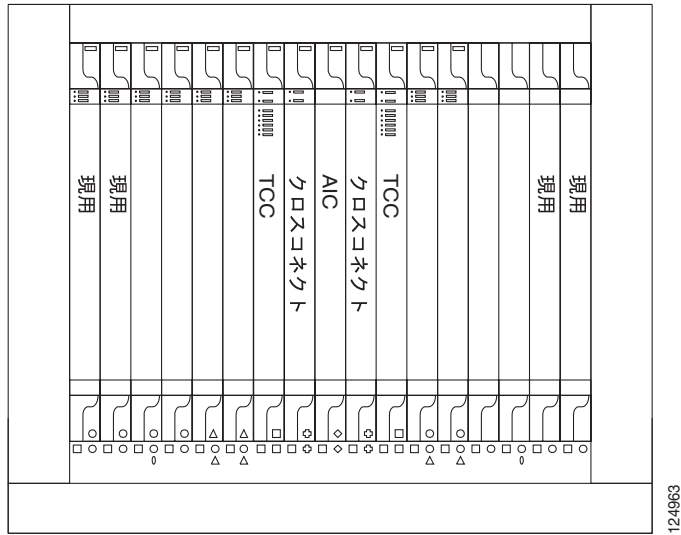
図 7-4 EIA タイプによる非保護の高密度電気回路カードのスキーム
