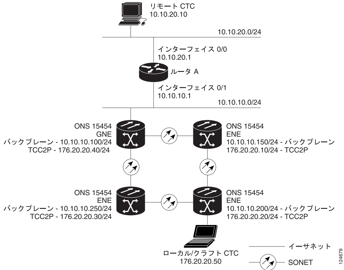
図 13-16 IP のシナリオ 9 : 同一サブネット上の ONS 15454 GNE および ENE (セキュア モードが有効な場合)
