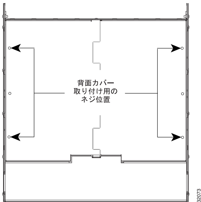
図 1-11 バックプレーン カバーの取り付け
