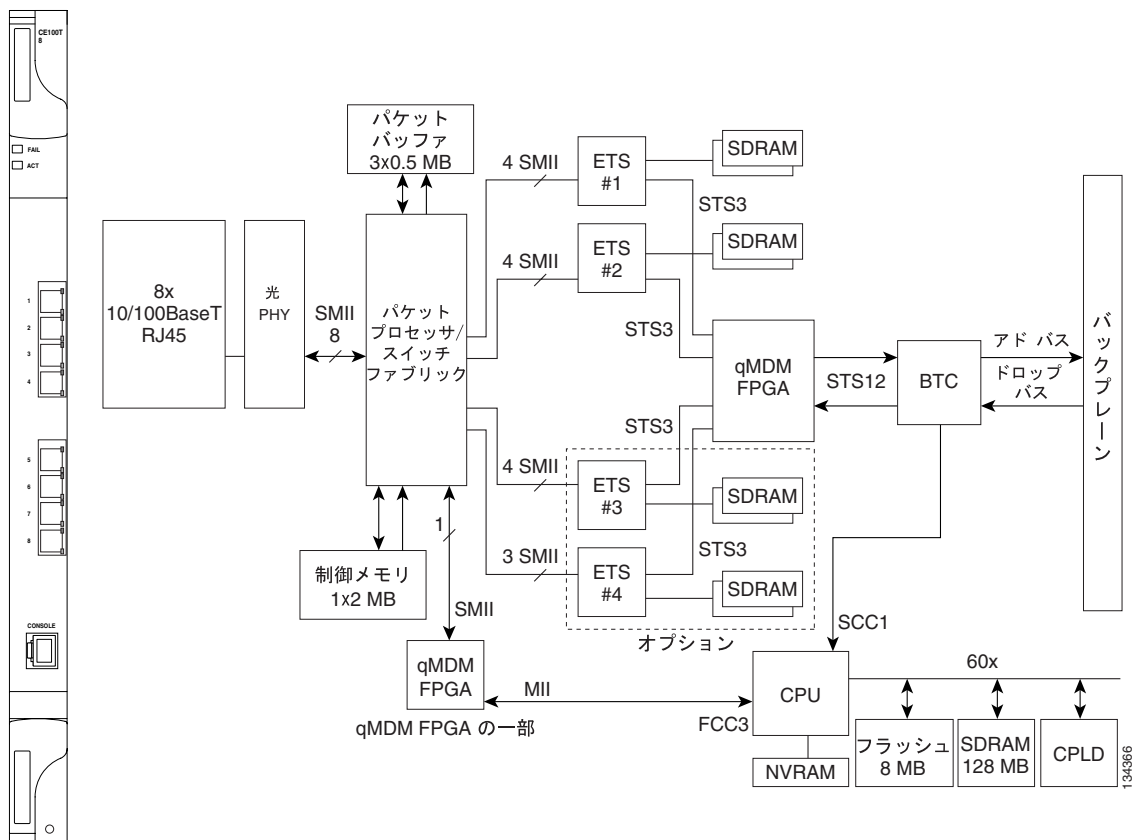
図 5-9 CE-100T-8 カードの前面プレートとブロック図
