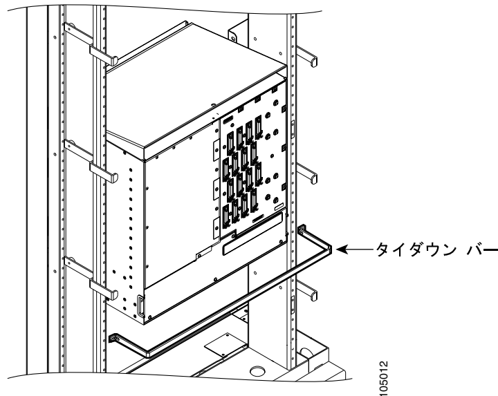
図 1-27 タイダウンバー
