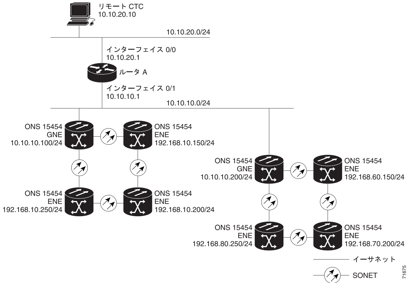
図 13-13 IP のシナリオ 7 : ENE が複数のリングにある ONS 15454 SOCKS プロキシ サーバ
