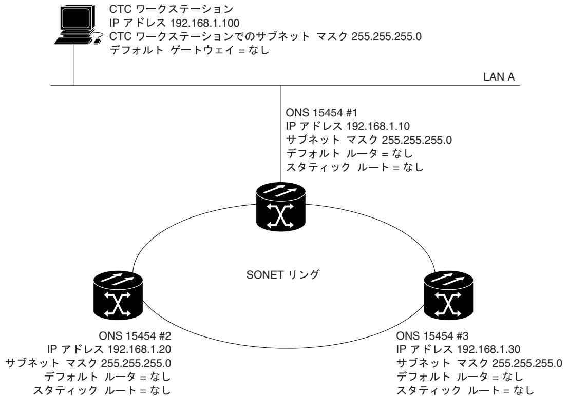
図 13-3 IP のシナリオ 3: プロキシ ARP の使用
