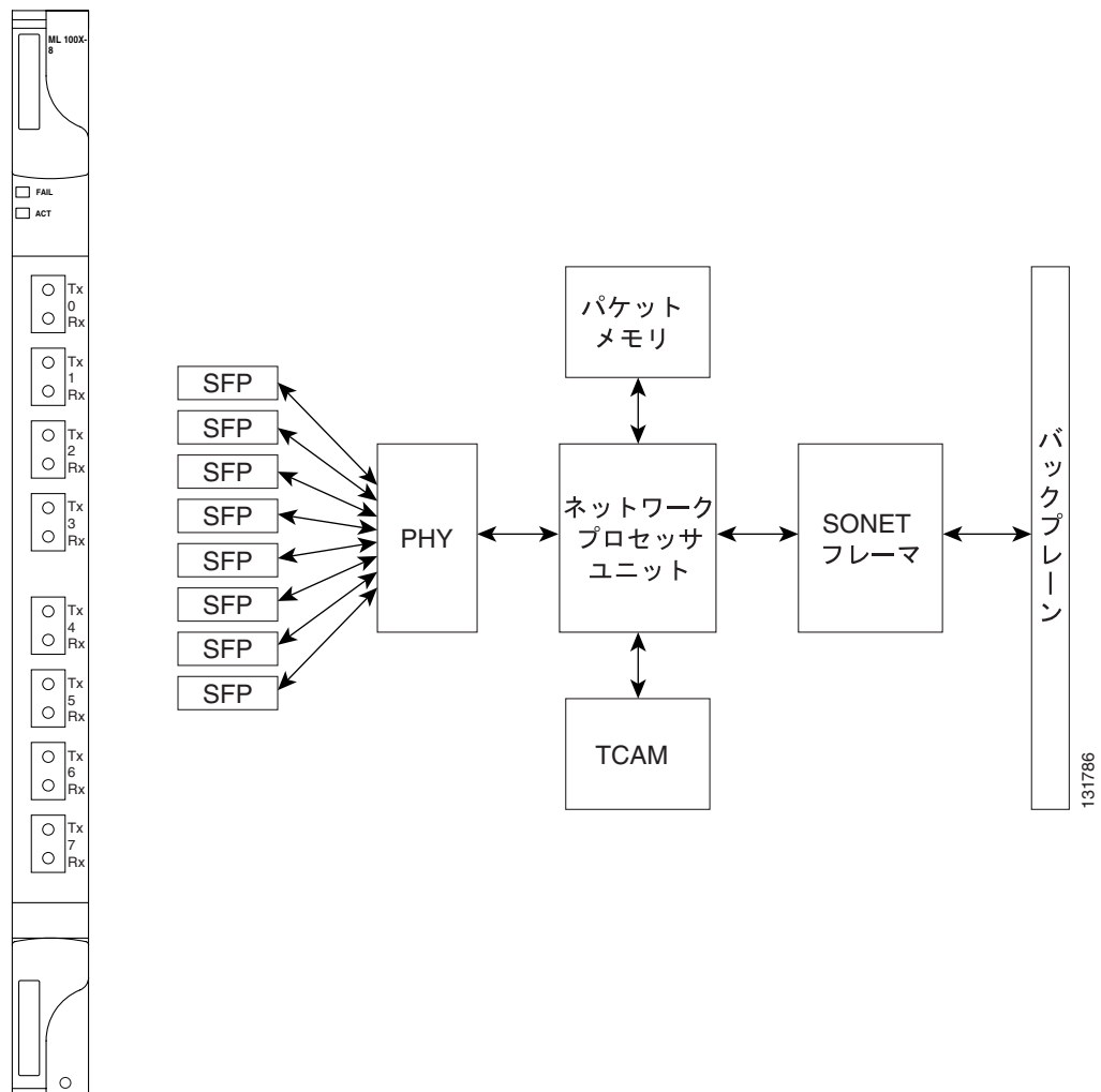
図 5-7 ML100X-8 カードの前面プレートとブロック図
