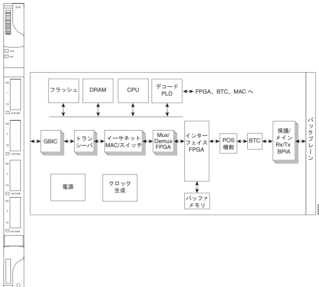
図 5-5 G1K-4 カードの前面プレートとブロック図
