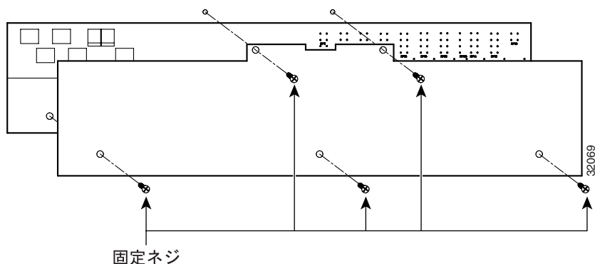
図 1-10 バックプレーン下部カバーの取り外し
