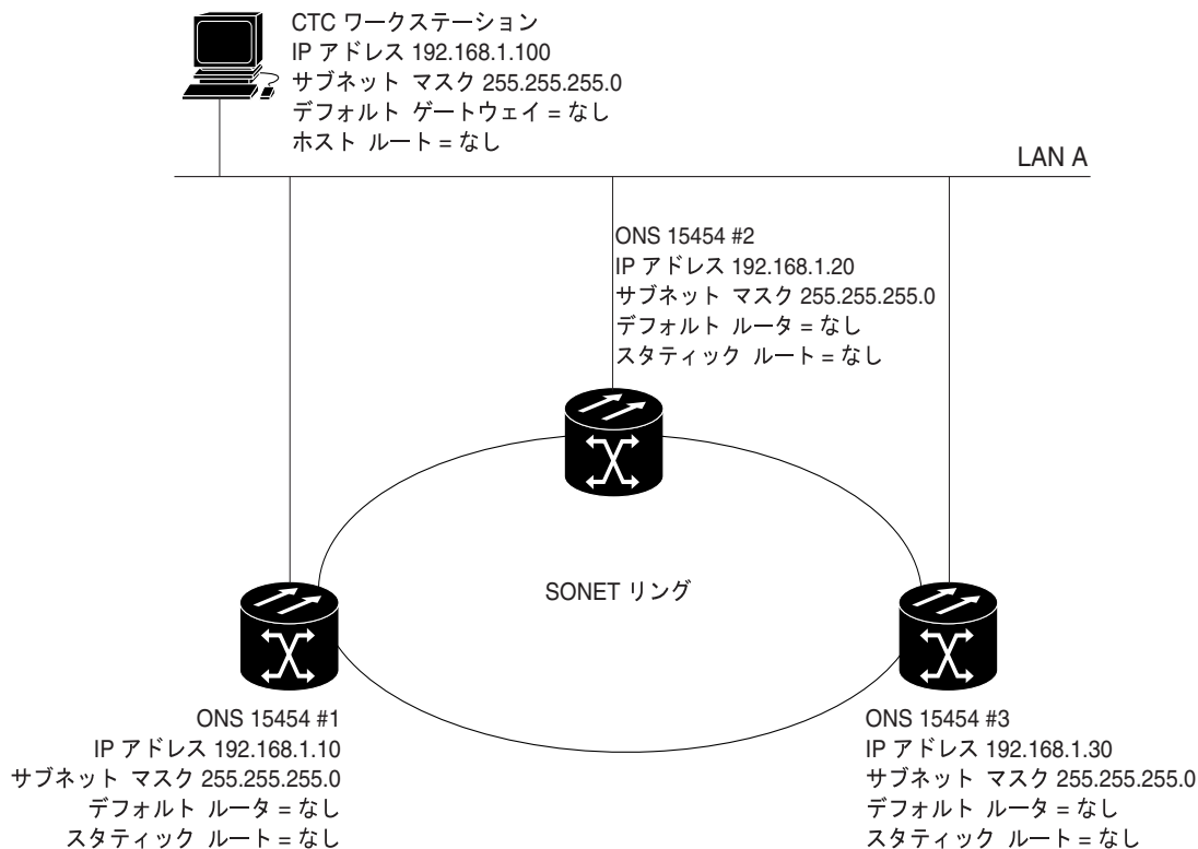
図 13-1 IP のシナリオ 1 : 同一サブネット上の CTC および ONS 15454
