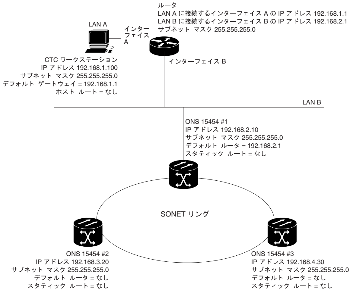
図 13-8 IP のシナリオ 6 : OSPF が有効な場合
