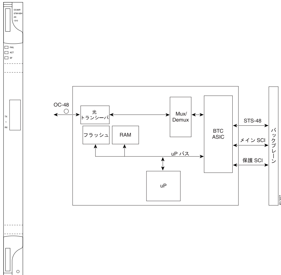
図 4-9 OC48 IR/STM16 SH AS 1310 カードの前面プレートとブロック図
