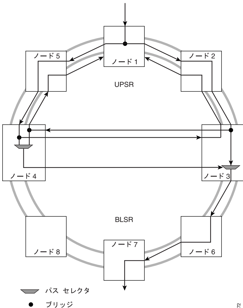
図 12-24 ONS 15454 UPSR/BLSR 統合型 DRI ハンドオフ
