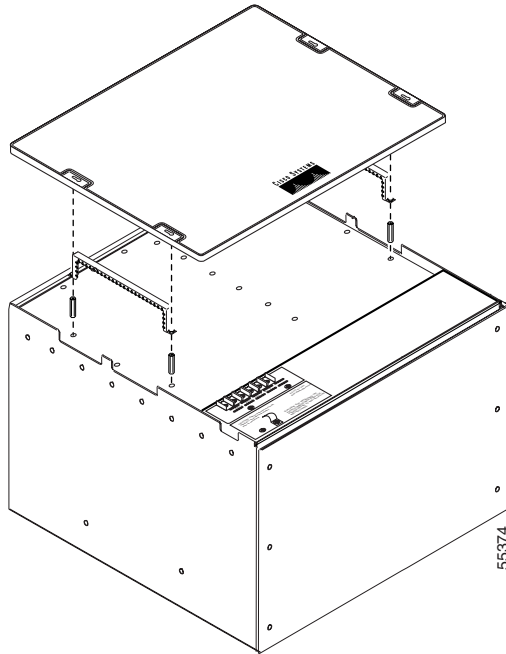
図 1-12 スペーサを使用したプラスチック製背面カバーの取り付け
