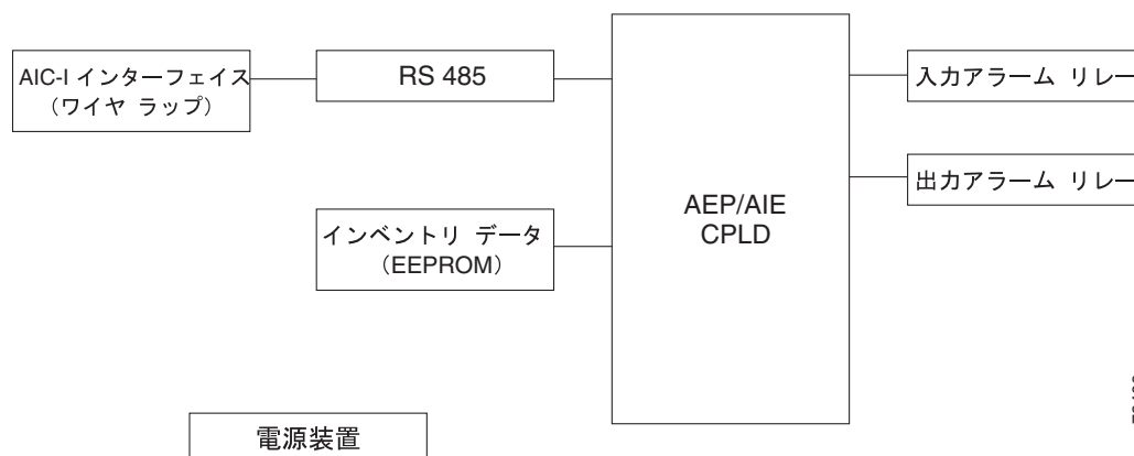
図 1-29 AEP のブロック図
