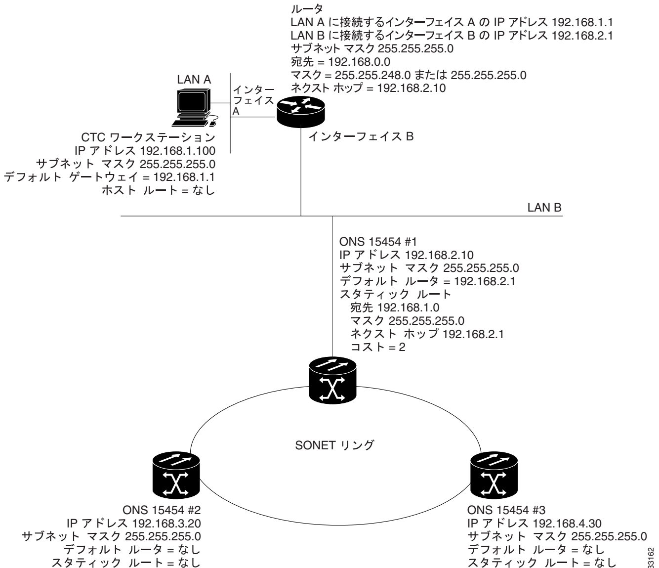
図 13-6 IP のシナリオ 5 : 宛先として使用される CTC コンピュータのスタティック ルート
