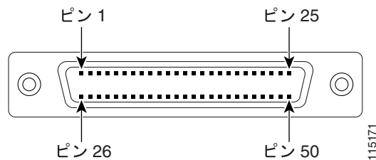
図 1-23 ケーブルのコネクタピン
