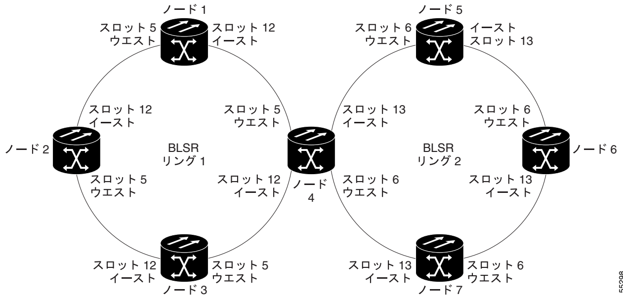
図 12-27 BLSR に従属する BLSR
