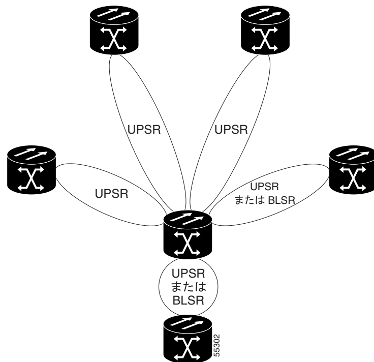
図 12-25 複数の従属リングのある ONS 15454
