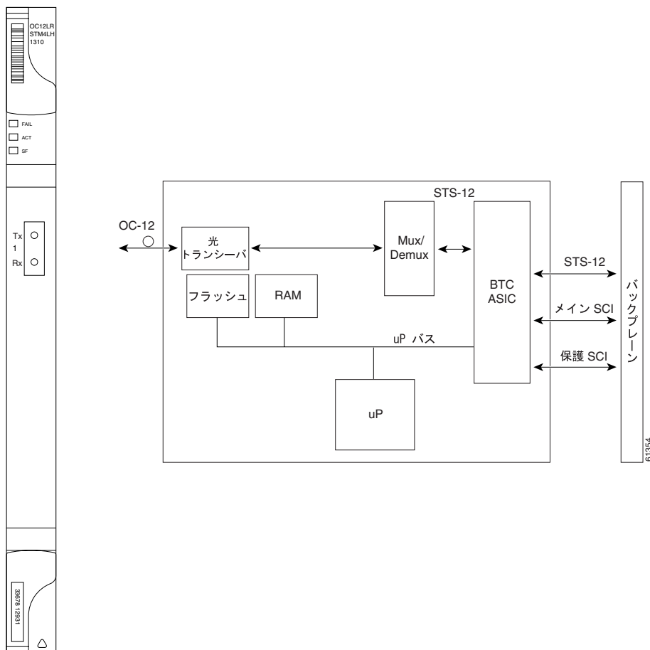
図 4-4 OC12 LR/STM4 LH 1310 カードの前面プレートとブロック図
