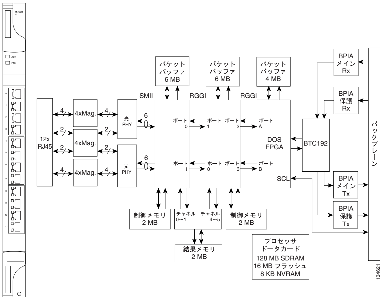
図 5-6 ML100T-12 カードの前面プレートとブロック図
