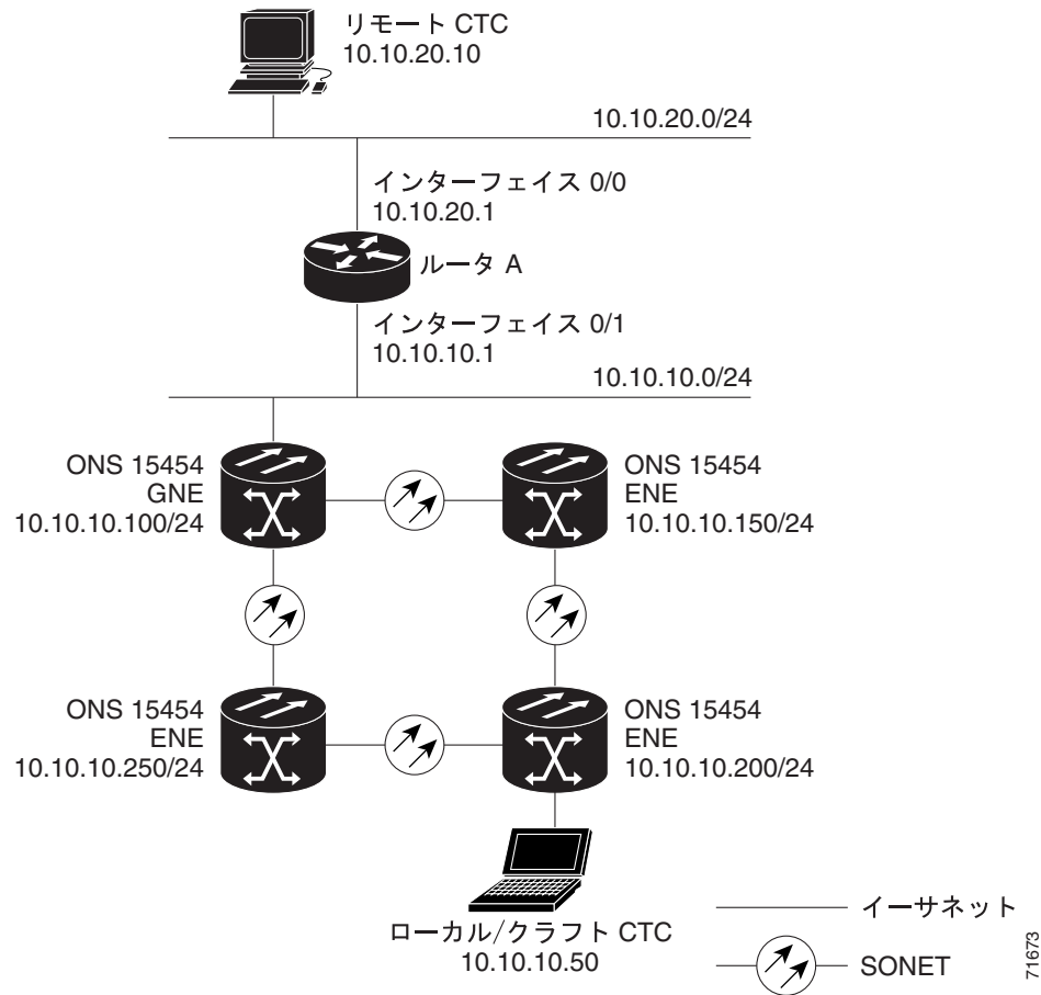
図 13-11 IP のシナリオ 7: 同一サブネット上に GNE と ENE が配置された ONS 15454 SOCKS プロキシサーバ
