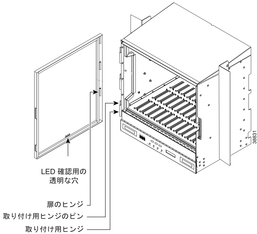
図 1-6 ONS 15454 の前面扉の取り外し
