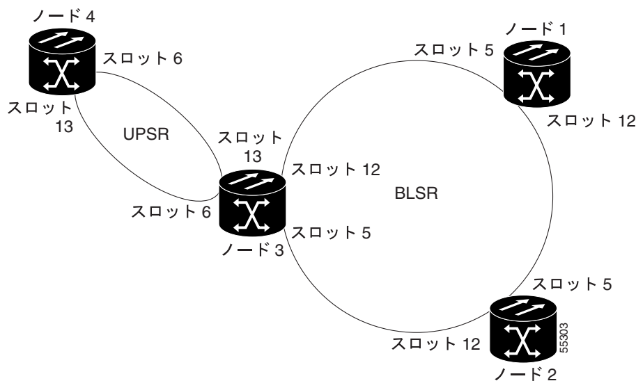
図 12-26 BLSR に従属する UPSR
