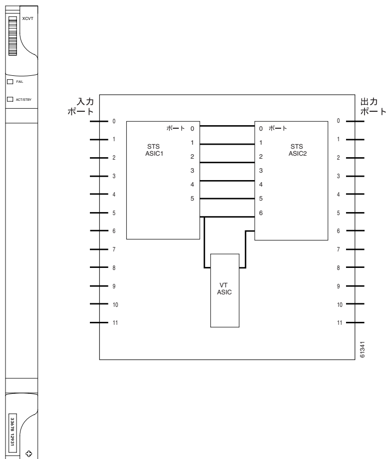
図 2-3 XCVT カードの前面プレートとブロック図
