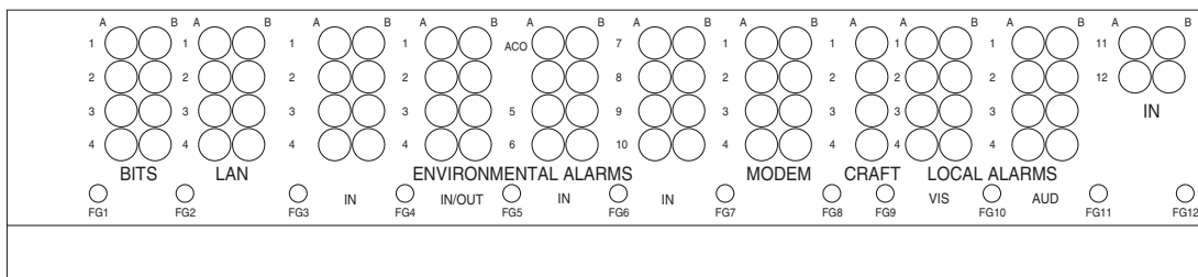
図 1-35 ONS 15454 バックプレーンのピン割り当て (Release 3.4 以上)
