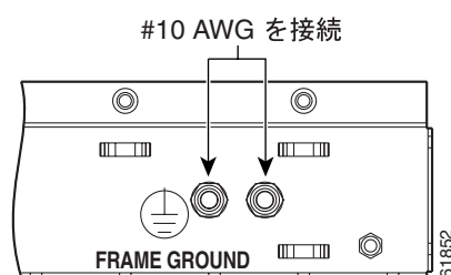
図 1-34 ONS 15454 バックプレーンのアース ポスト
