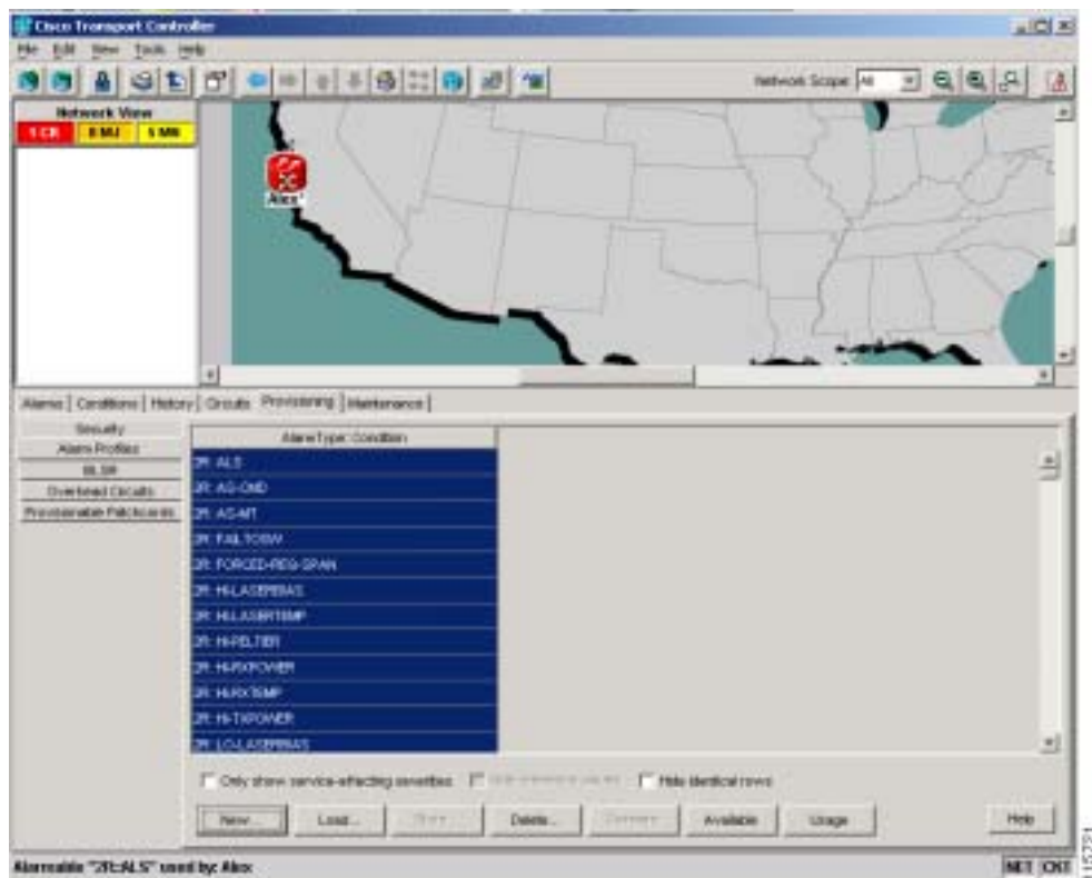
図 14-3 ネットワーク ビューの Alarm Profiles ウィンドウ
