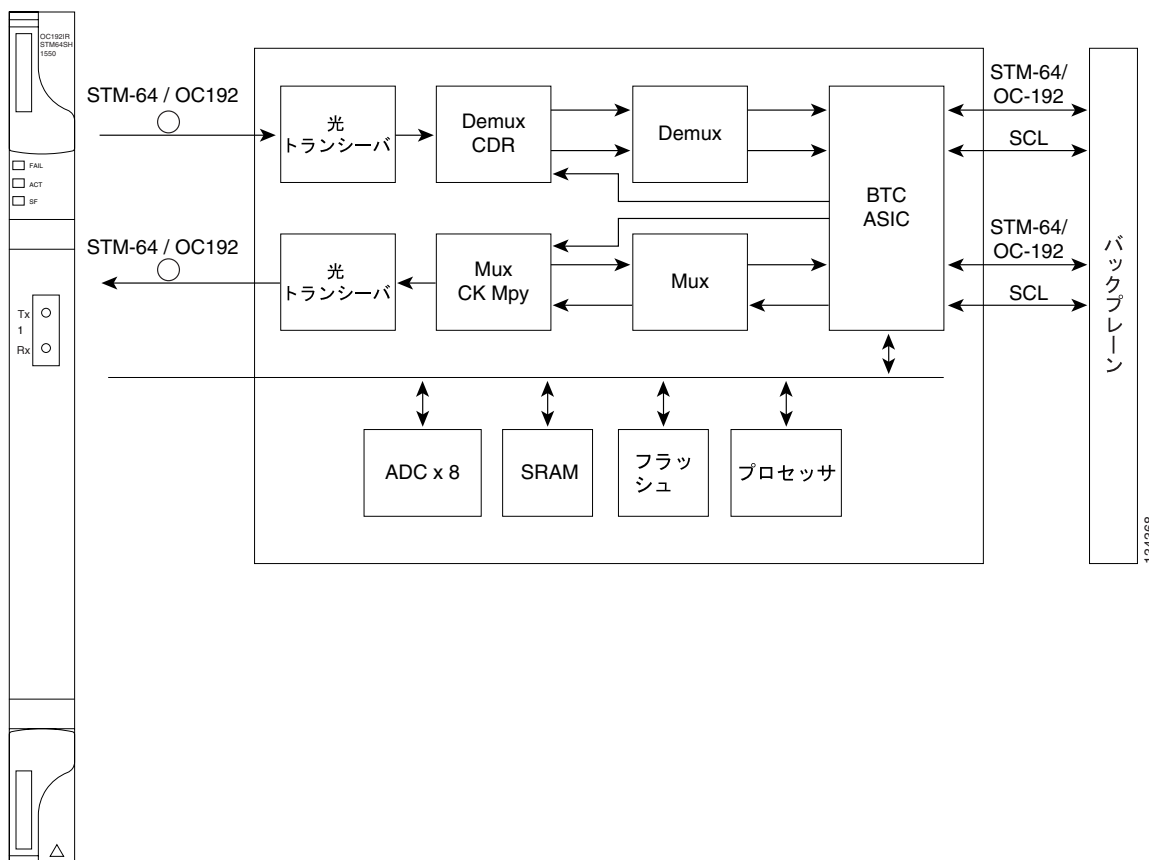
図 4-14 OC192 IR/STM64 SH 1550 カードの前面プレートとブロック図
