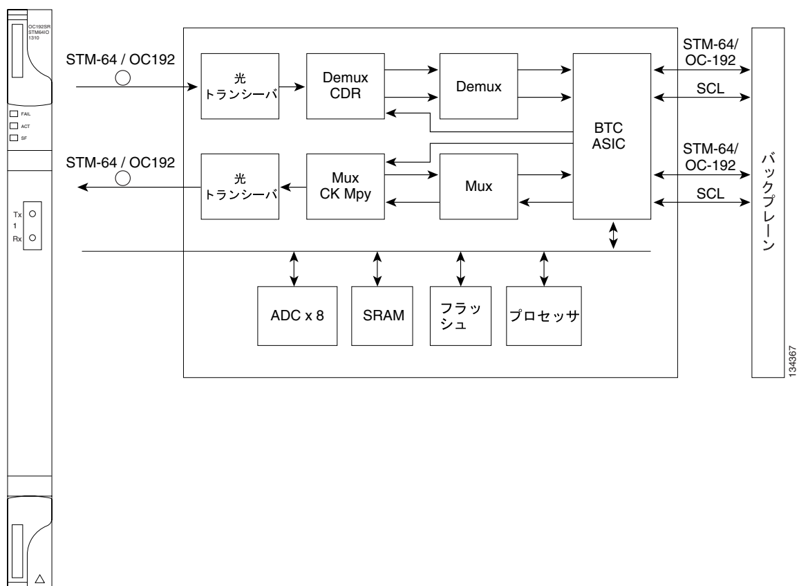
図 4-13 OC192 SR/STM64 IO 1310 カードの前面プレートとブロック図
