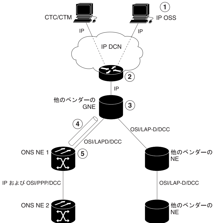
図 13-34 OSI/IP のシナリオ 3 : OSI/IP-over-CLNS トンネルのエンド ポイントが GNE にある場合
