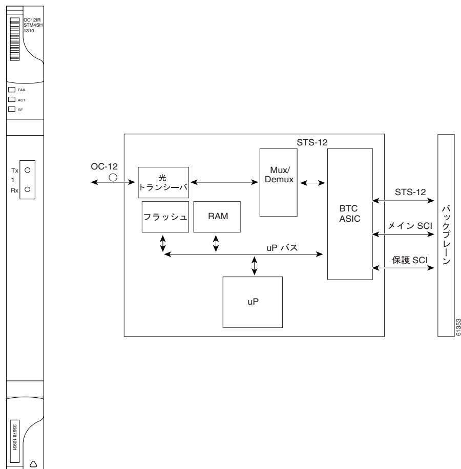
図 4-3 OC12 IR/STM4 SH 1310 カードの前面プレートとブロック図
