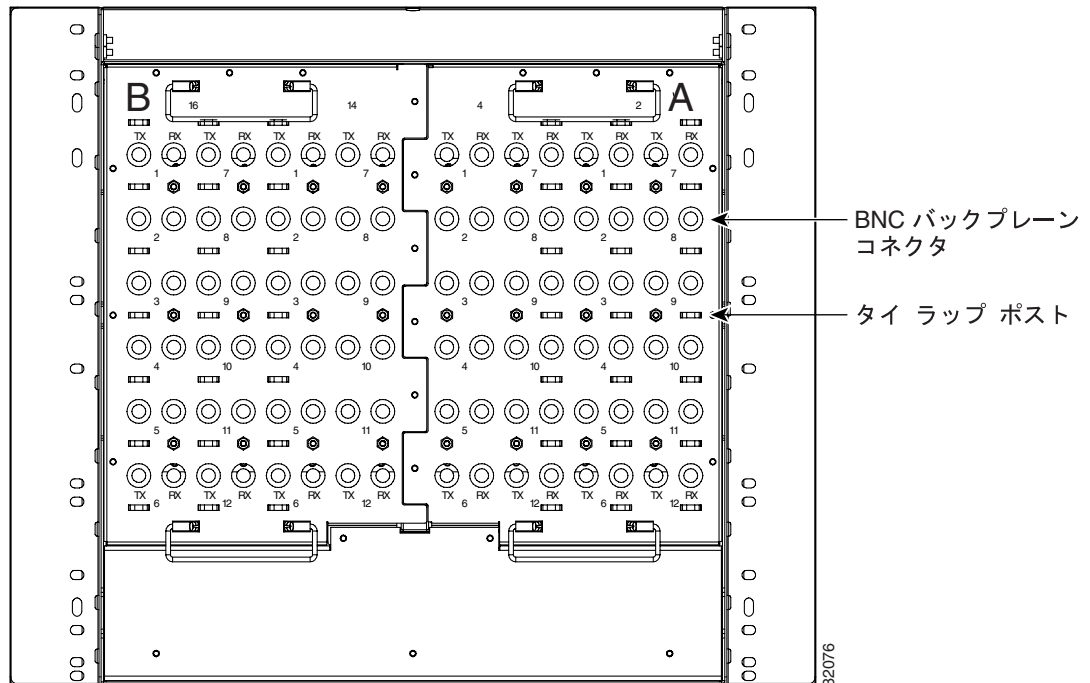
図 1-13 1:1 保護スキームで使用する BNC バックプレーン
