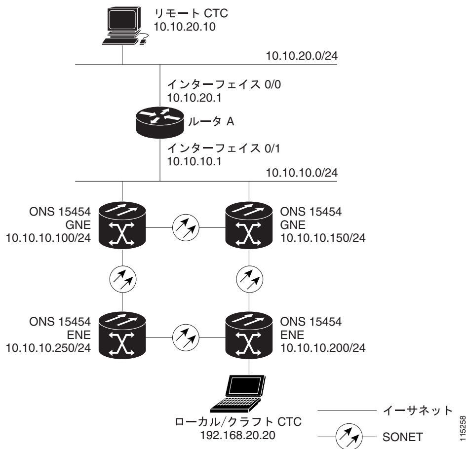
図 13-14 IP のシナリオ 8 : 同一サブネット上のデュアル GNE
