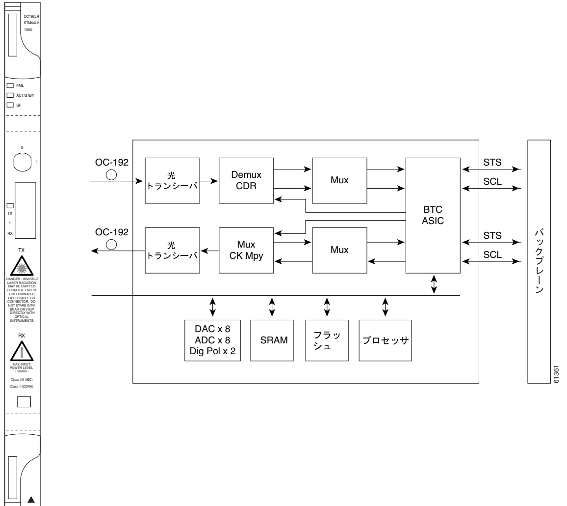
図 4-15 OC192 LR/STM64 LH 1550 ( 15454-OC192LR1550 ) カードの前面プレートとブロック図
