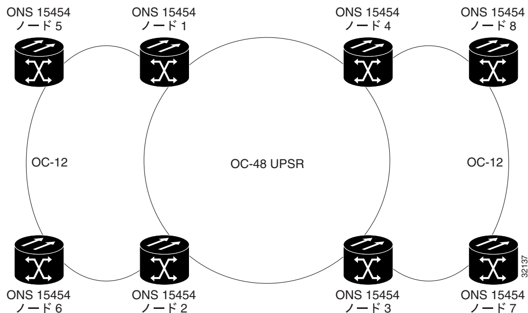
図 12-30 PPMN 仮想リング
