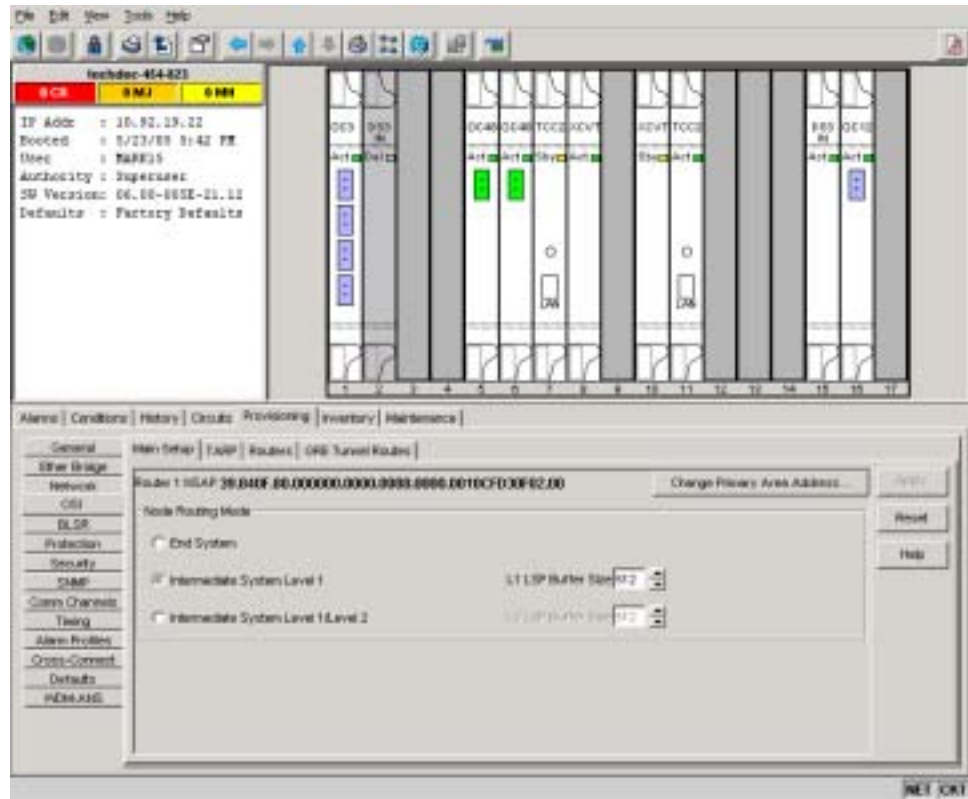
図 13-21 OSI の主要な設定
