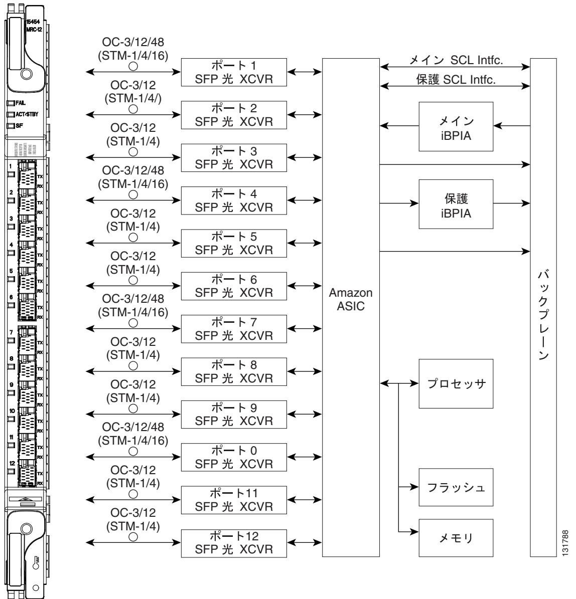
図 4-21 15454_MRC-12 カードの前面プレートとブロック図
