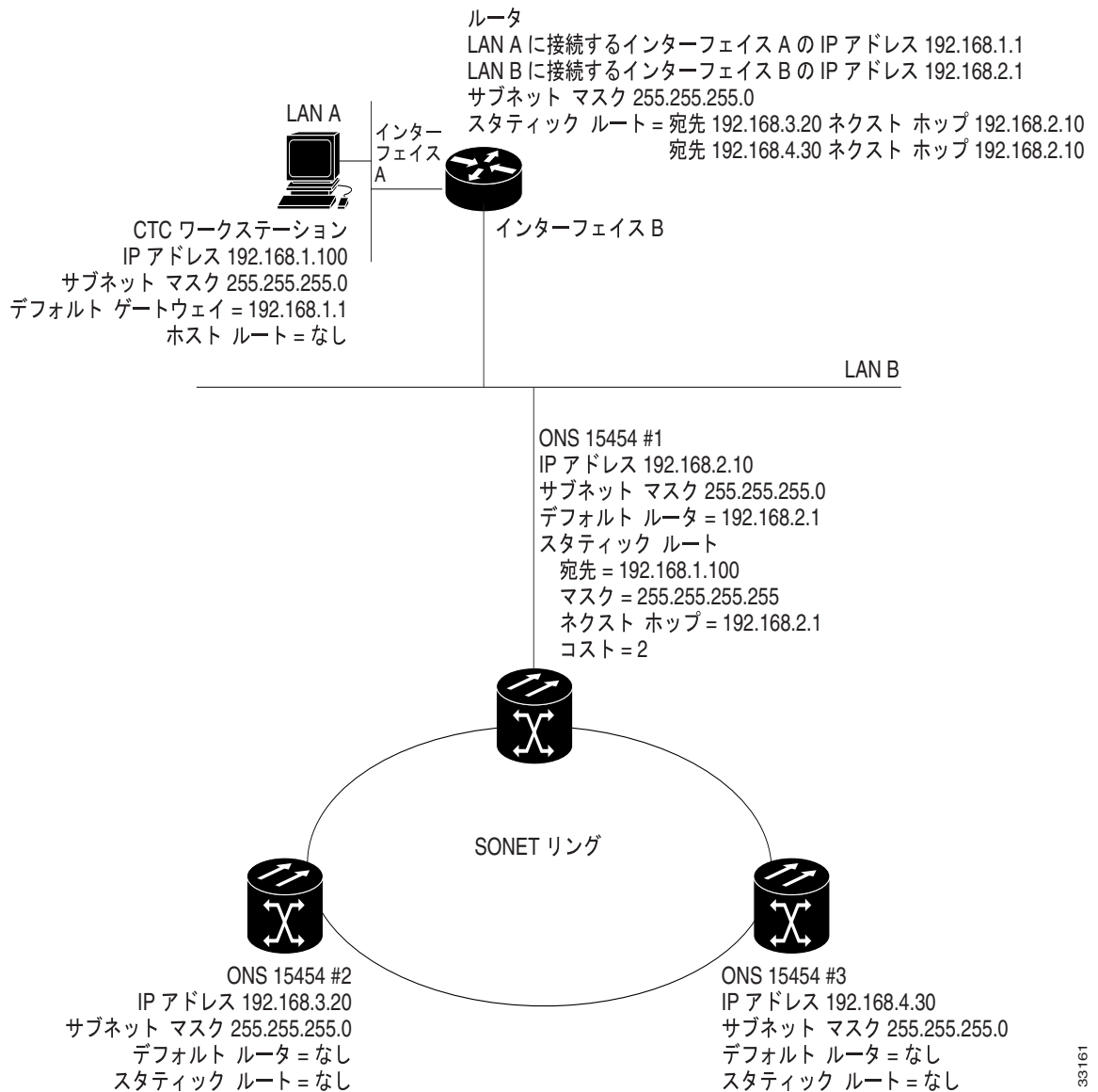
図 13-9 IP のシナリオ 6 : OSPF が有効でない場合
