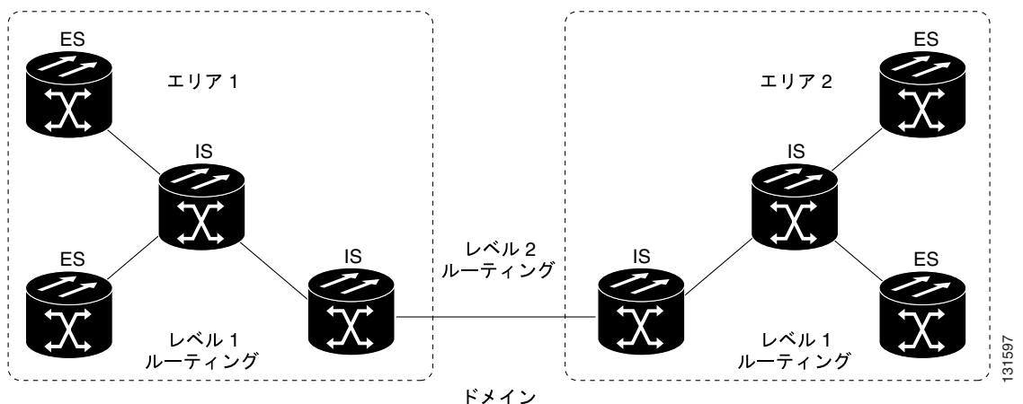
図 13-22 レベル 1 およびレベル 2 の OSI ルーティング
