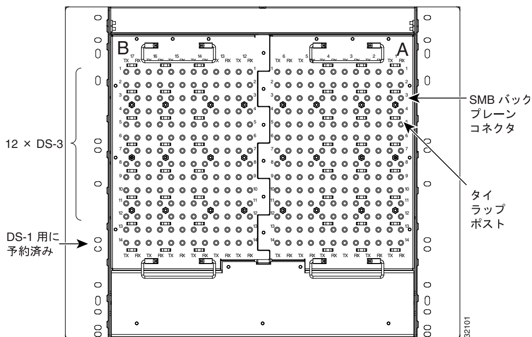
図 1-18 SMB EIA のバックプレーン
