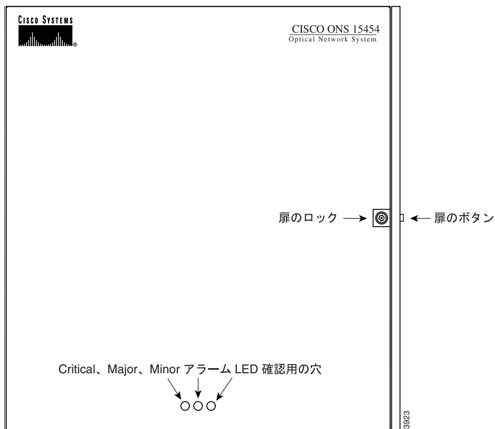
図 1-3 ONS 15454 の前面扉
