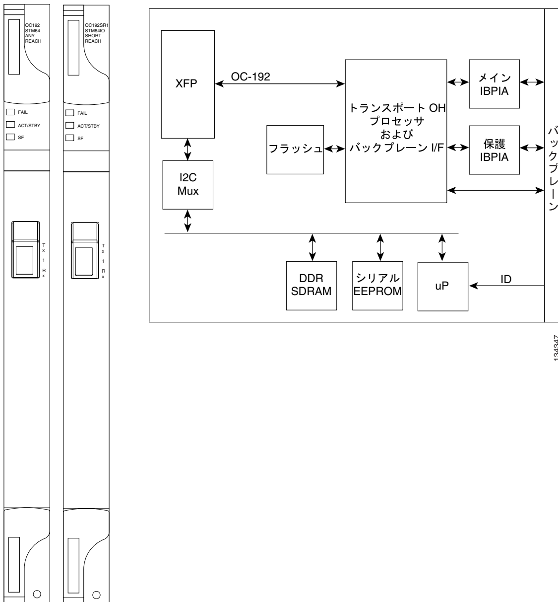
図 4-22 OC192SR1/STM64IO Short Reach および OC192/STM64 Any Reach カードの前面プレートとブロック図
