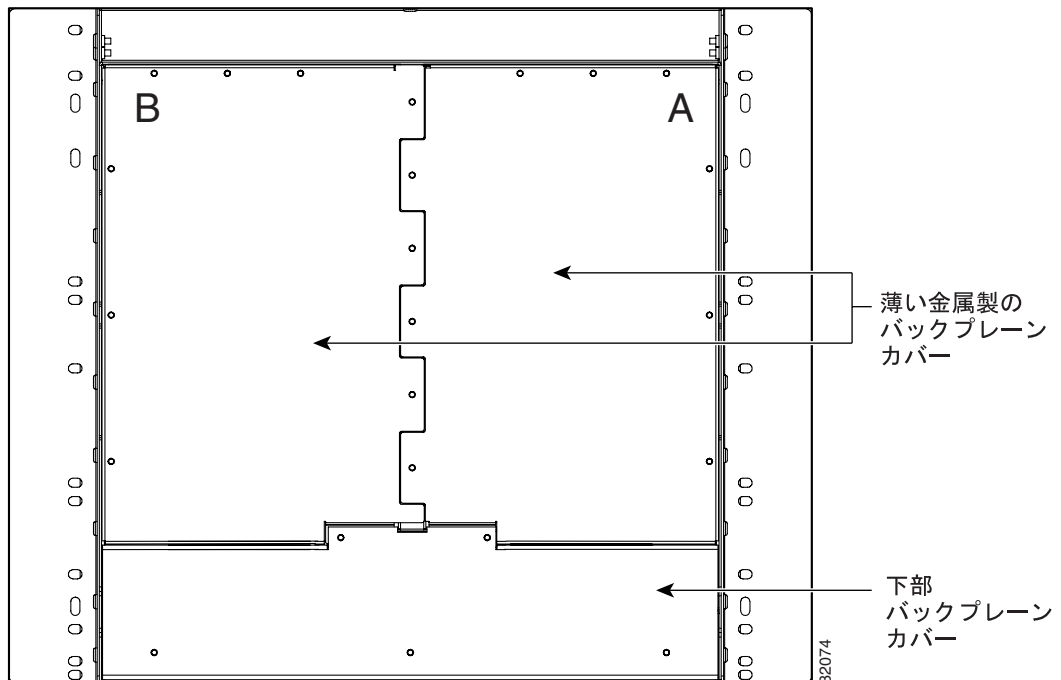
図 1-9 バックプレーンカバー
