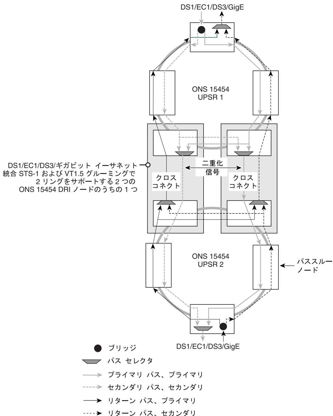
図 12-22 ONS 15454 統合型 UPSR デュアル リング相互接続
