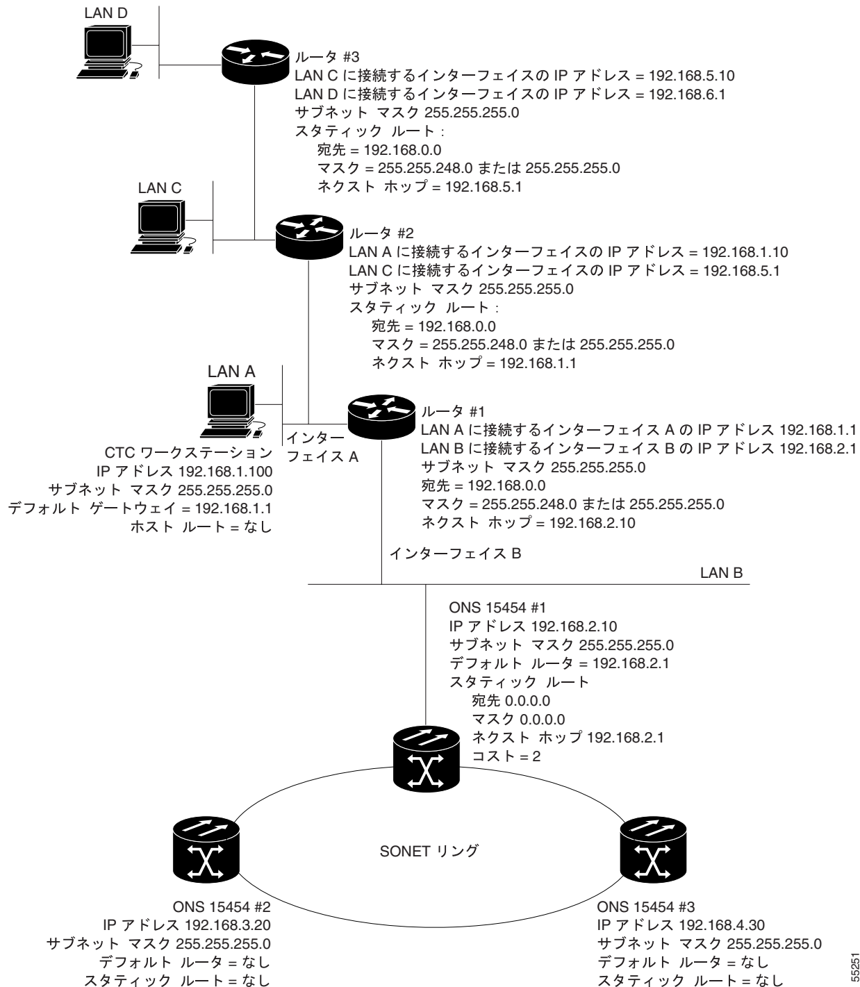
図 13-7 IP のシナリオ 5 : 複数の LAN 宛先のスタティック ルート
