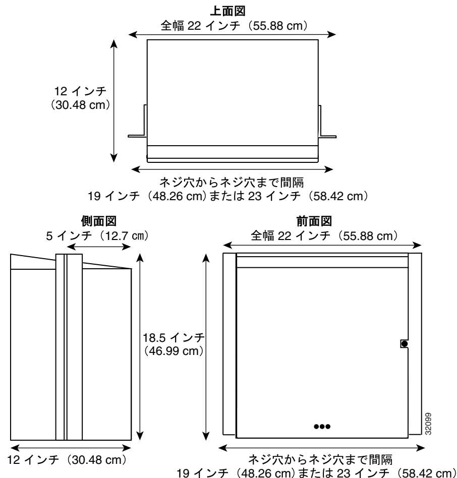
図 1-1 Cisco ONS 15454 ANSI の寸法
