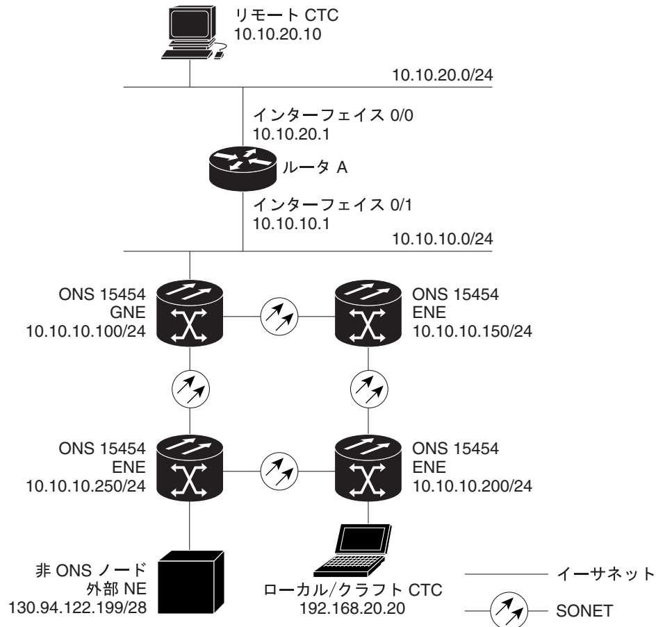
図 13-19 ENE イーサネット ポートへの外部ノード接続
