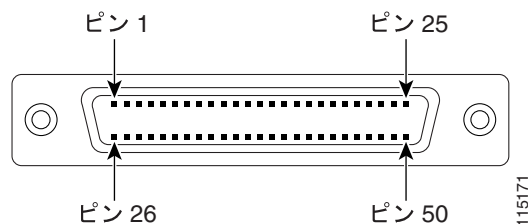
図 1-24 ケーブルのコネクタ ピン
