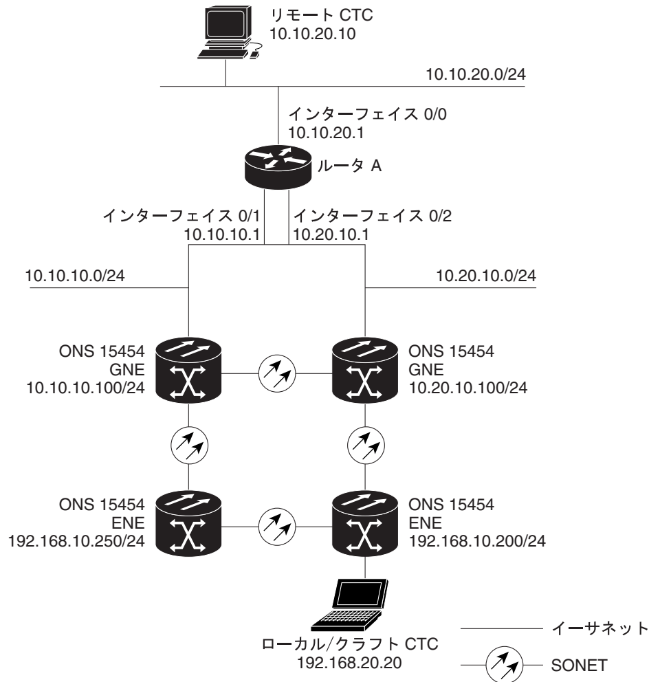
図 13-15 IP のシナリオ 8 : 異なるサブネット上のデュアル GNE
