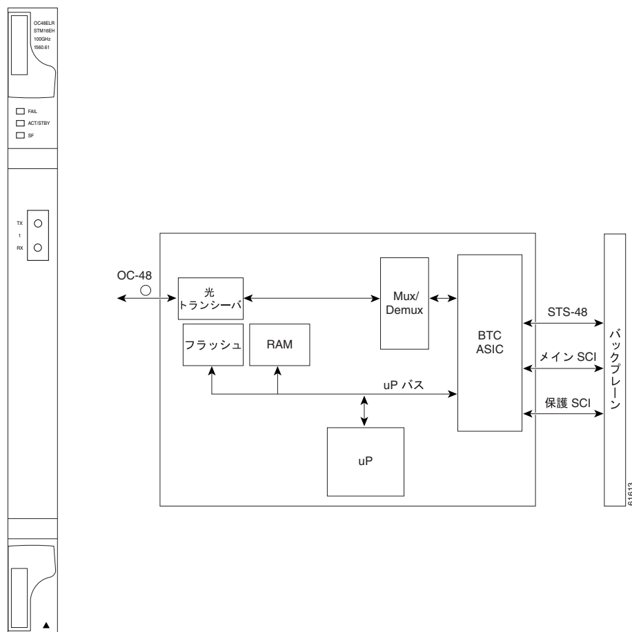
図 4-11 OC48 ELR/STM16 EH 100 GHz カードの前面プレートとブロック図
