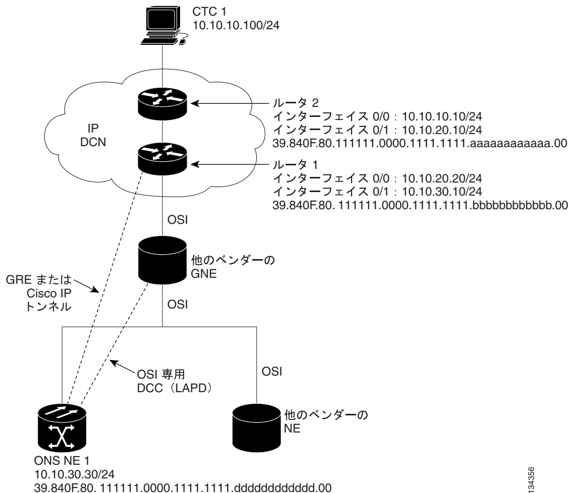
図 13-29 IP-over-CLNS トンネルのシナリオ 2 : ONS ノードからルータへ
