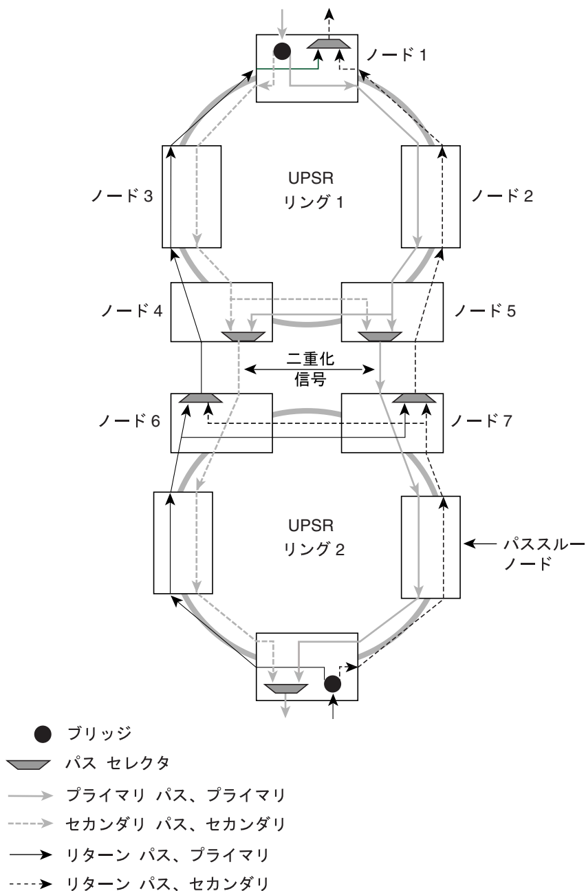
図 12-21 ONS 15454 従来型 UPSR デュアル リング相互接続
