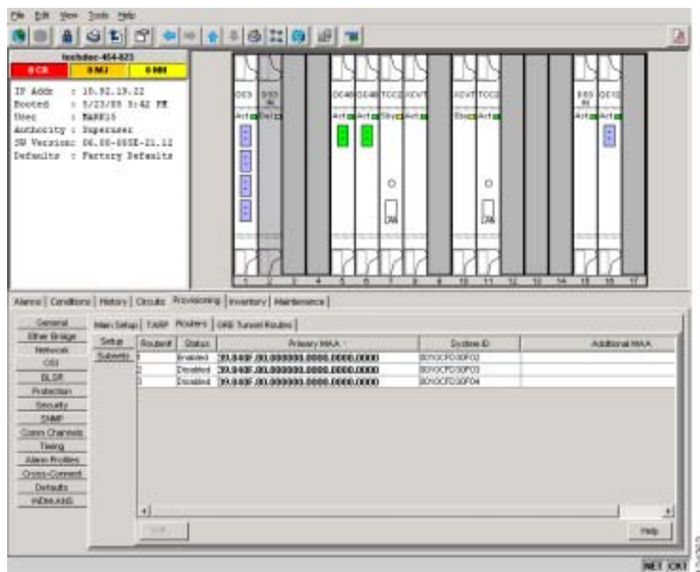
図 13-26 OSI ルータのプロビジョニング
