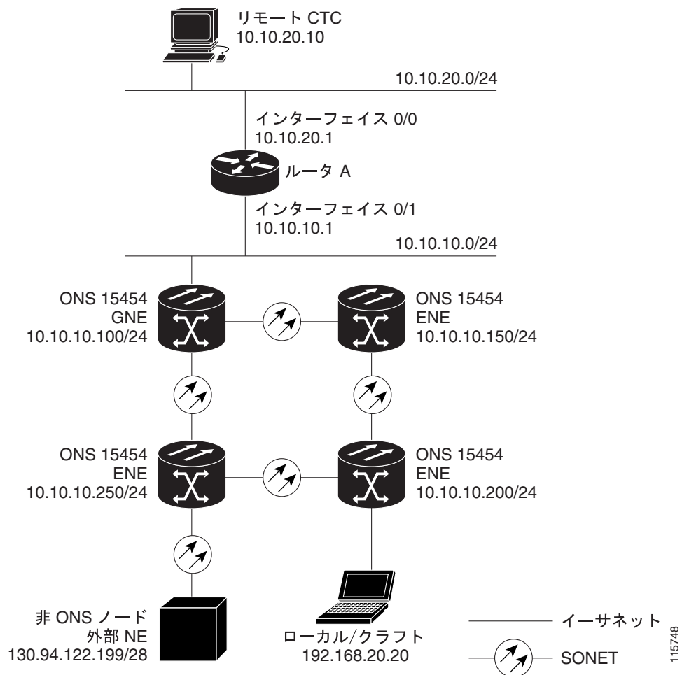
図 13-18 外部で終端する場合のプロキシ トンネルおよびファイアウォールトンネル
