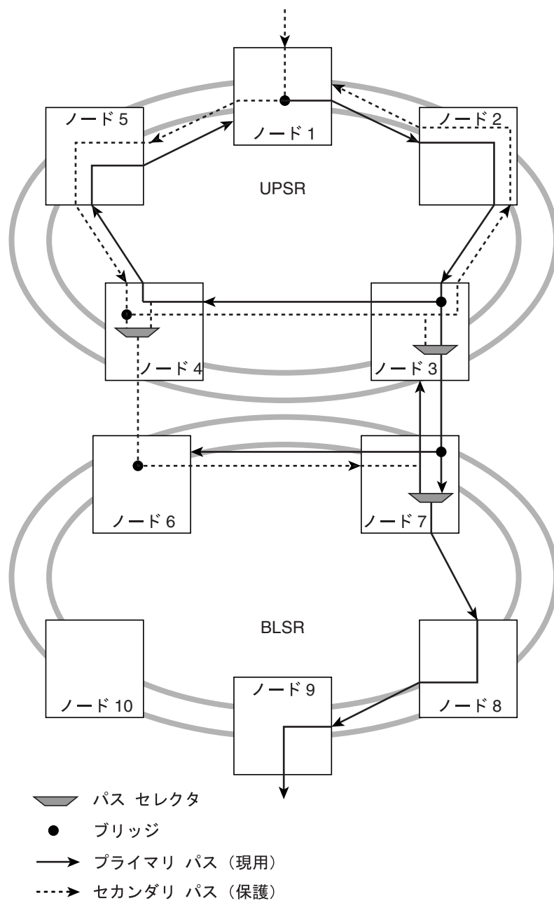
図 12-23 ONS 15454 UPSR/BLSR 従来型 DRI ハンドオフ
