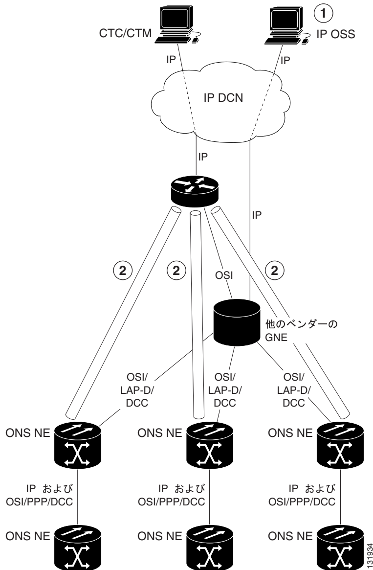
図 13-35 OSI/IP のシナリオ 4 : 複数の ONS DCC エリア
