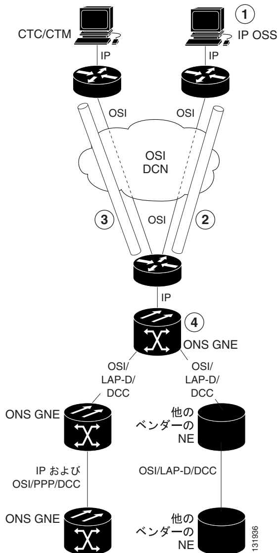
図 13-37 OSI/IP のシナリオ 6 : IP OSS、OSI DCN、ONS GNE、OSI DCC、および他のベンダーの ENE
