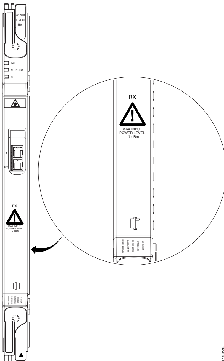
図 4-18 OC192 LR/STM64 LH 1550 (15454-OC192-LR2) 前面プレートの拡大図
