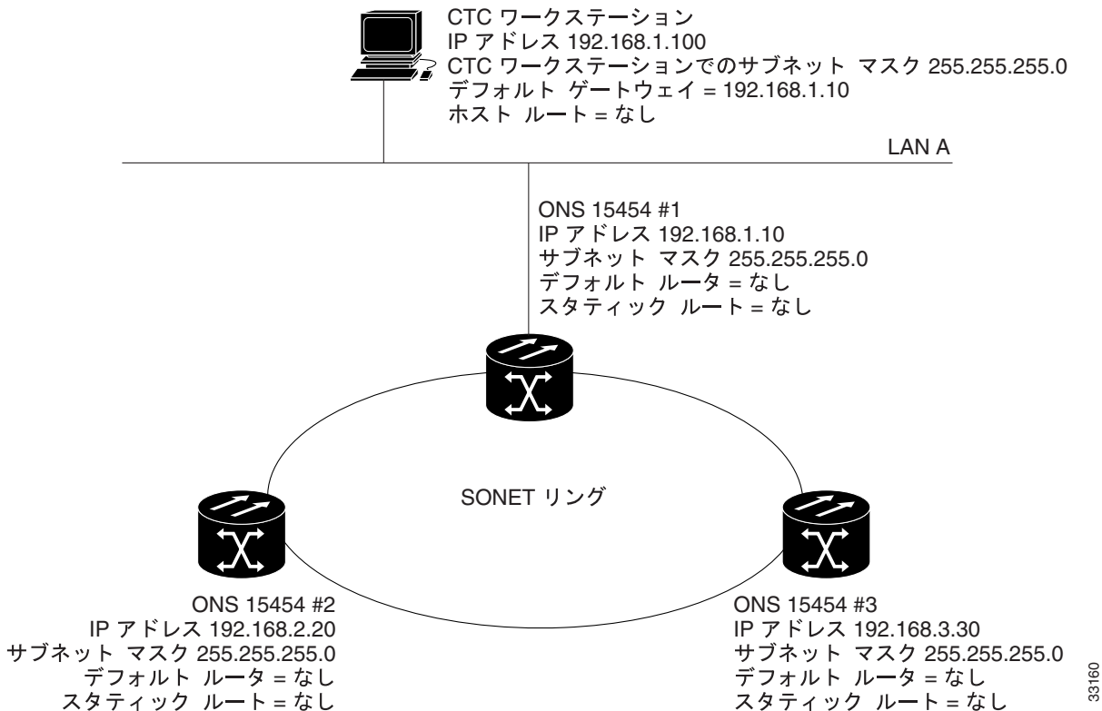
図 13-5 IP のシナリオ 4 : CTC コンピュータ上のデフォルト ゲートウェイ
