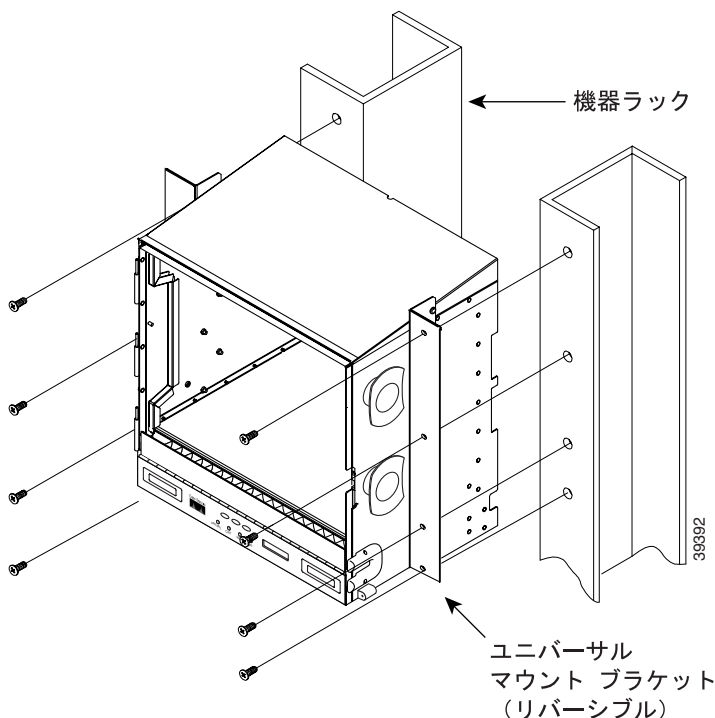
図 1-2 ONS 15454 のラックへの取り付け
