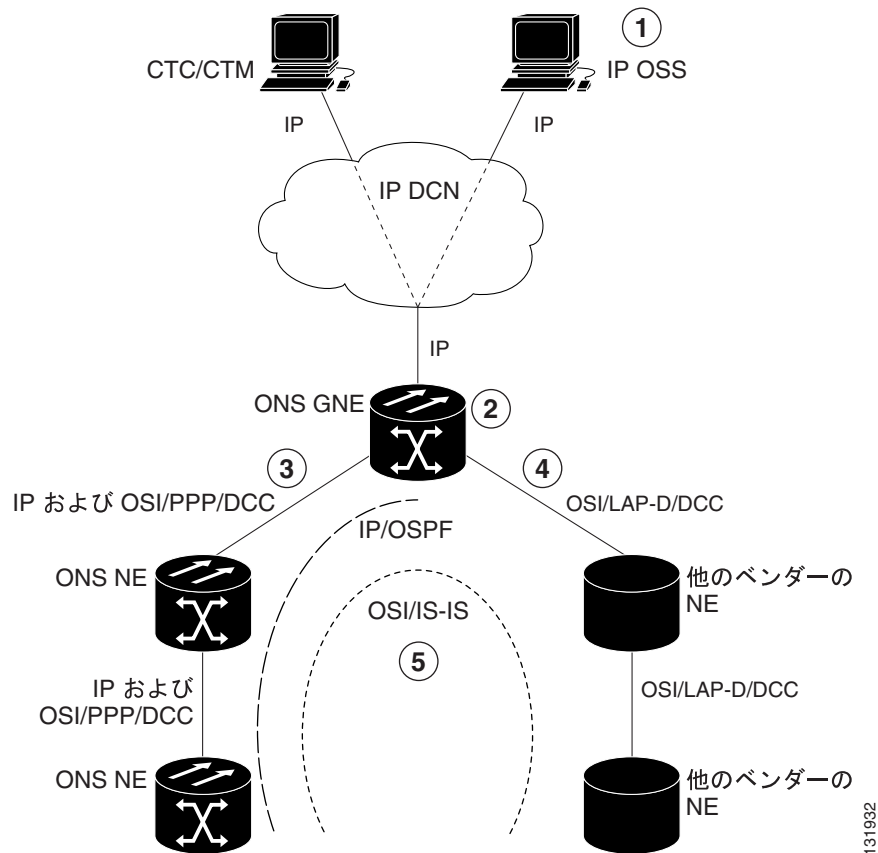
図 13-32 OSI/IP のシナリオ 2 : IP OSS、IP DCN、ONS GNE、OSI DCC、および他のベンダーの ENE
