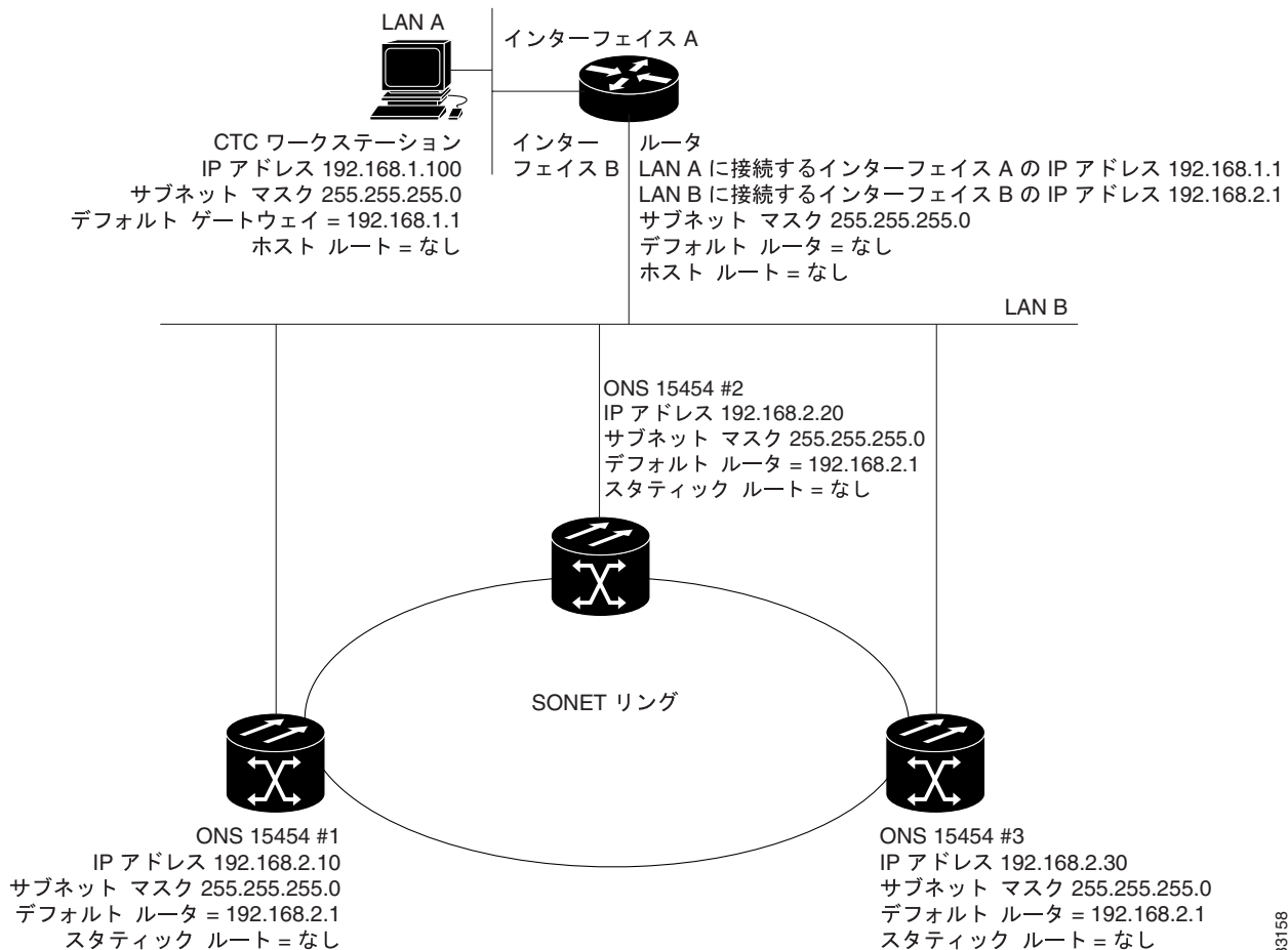
図 13-2 IP のシナリオ 2 : ルータに接続された CTC および ONS 15454 ノード
