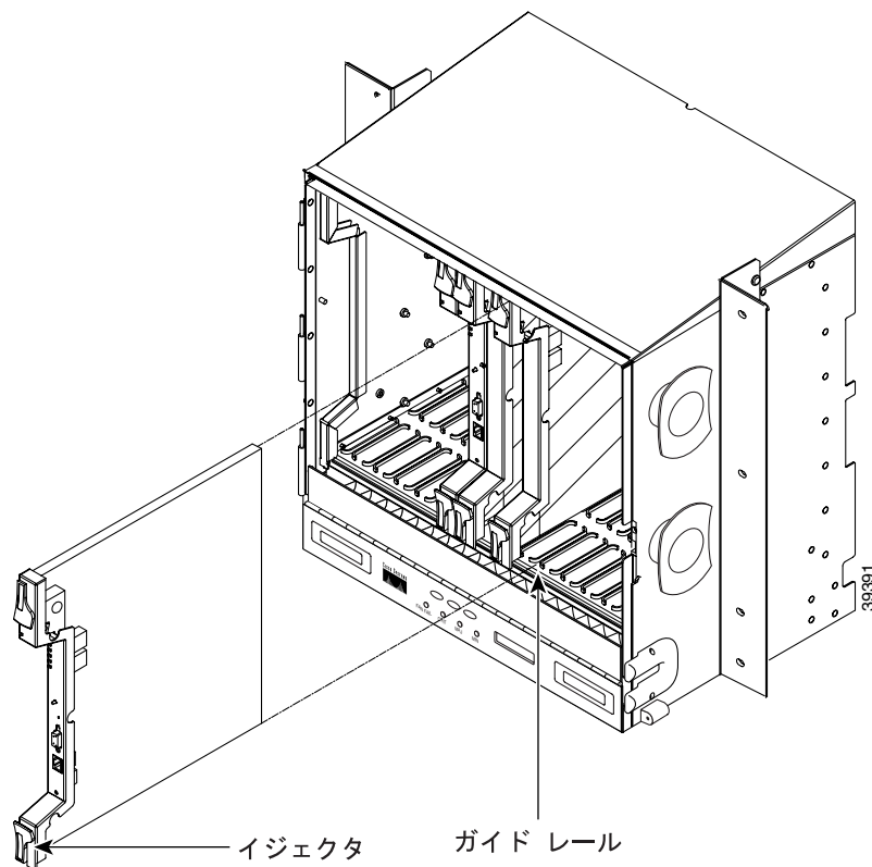
図 1-37 ONS 15454 へのカードの取り付け
