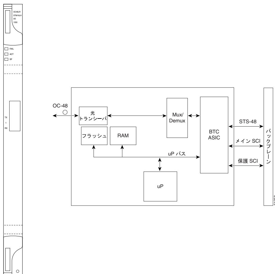
図 4-10 OC48 LR/STM16 LH AS 1550 カードの前面プレートとブロック図
