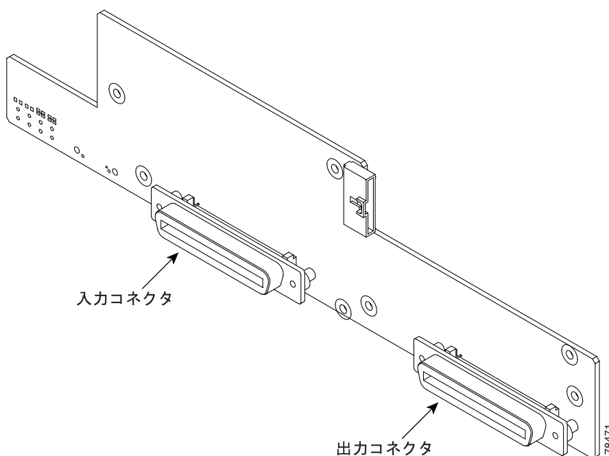
図 1-28 AEP プリント基板アセンブリ
