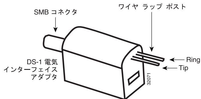
図 1-22 DS-1 電気インターフェイス アダプタ (バラン)
