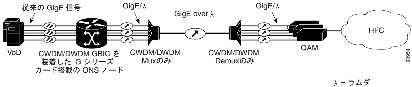
図 5-12 ケーブルネットワークでの CWDM/DWDM GBIC 搭載 G シリーズの使用
