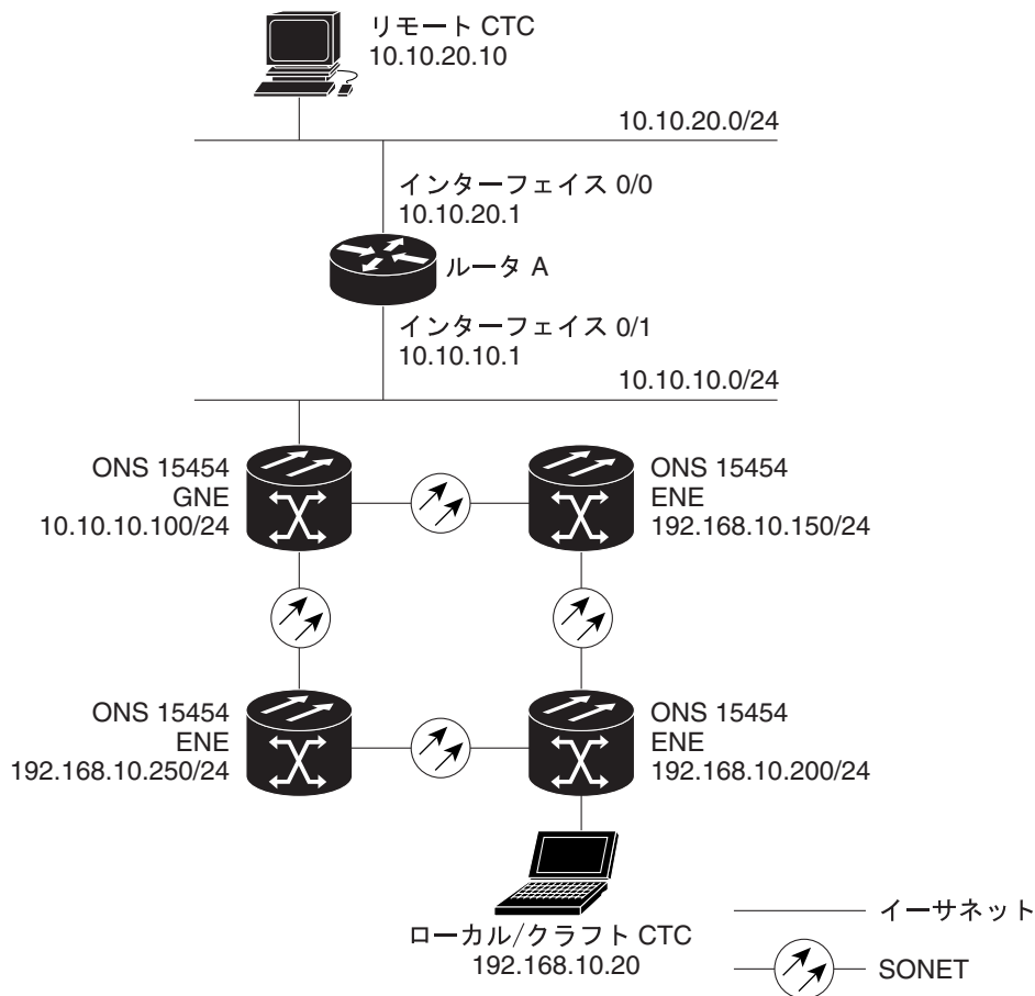
図 13-12 IP のシナリオ 7:異なるサブネット上に GNE と ENE が配置された ONS 15454 SOCKS プロキシサーバ
