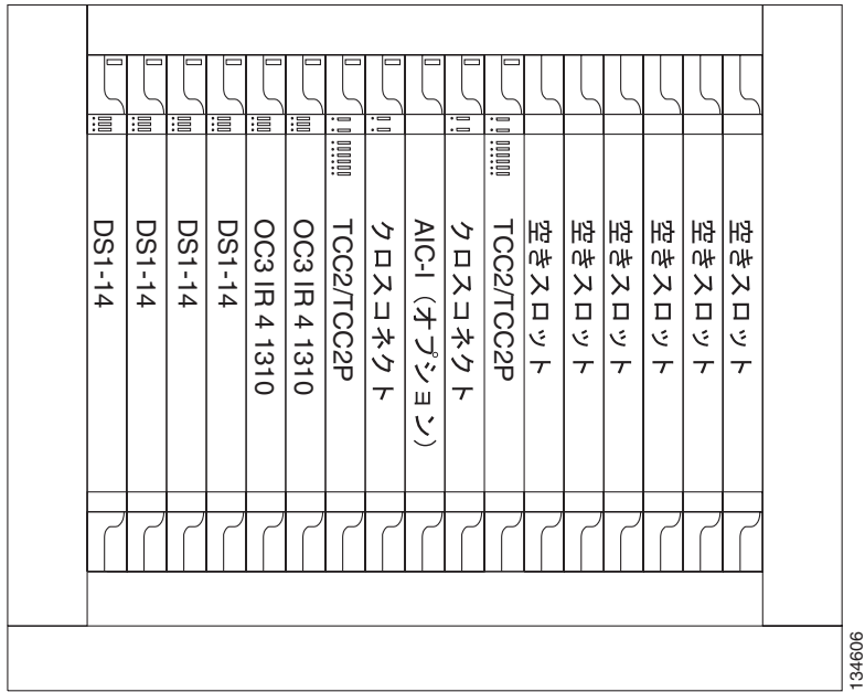
図 12-16 図 12-15 の OC-3 UPSR 例におけるノード ID 0 のレイアウト
