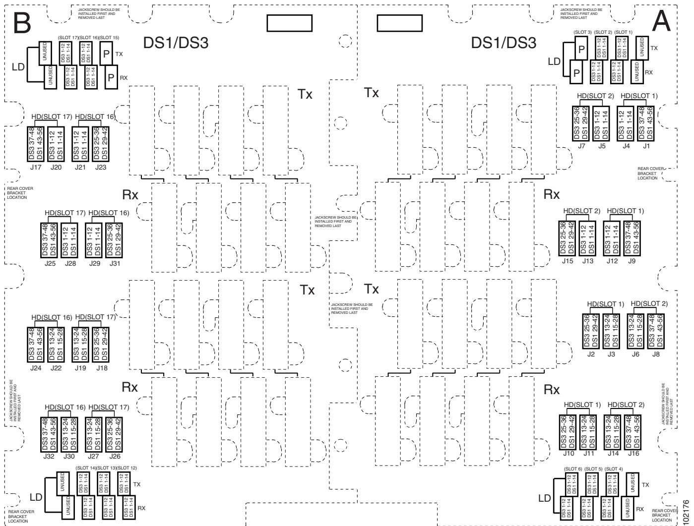
図 1-20 UBIC-V のスロット指定
