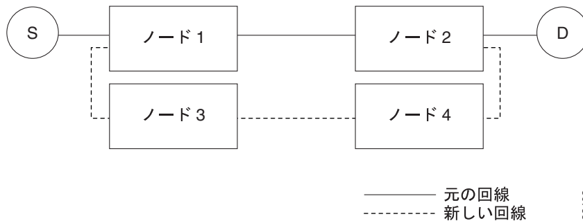
図 11-22 デュアル ロールによる異なるノードへの再ルーティング
