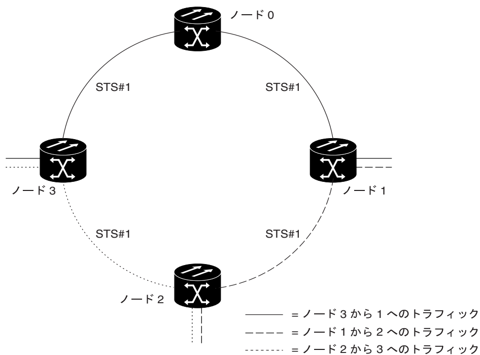
図 12-7 BLSR 帯域幅の再使用
