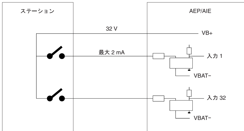
図 1-31 アラーム入力の回路図
