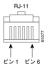
図 2-10 RJ-11 コネクタ
