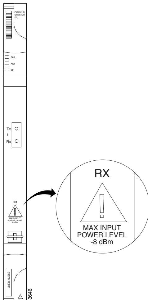
図 4-19 OC192 LR/STM64 LH ITU 15xx.xx カードの前面プレート
