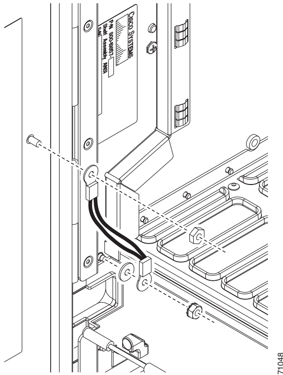
図 1-5 ONS 15454 の前面扉のアースストラップ
