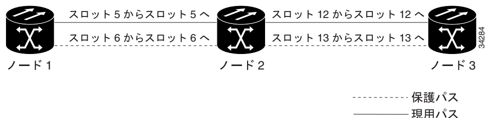
図 12-28 リニア (ポイントツーポイント) ADM 構成
