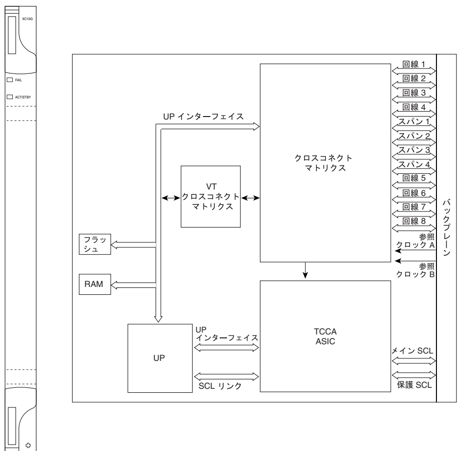
図 2-5 XC10G カードの前面プレートとブロック図
