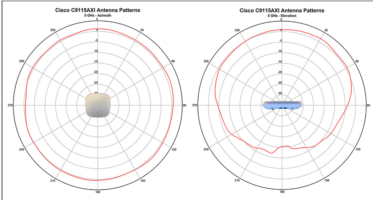
図 1. アンテナ放射パターン
