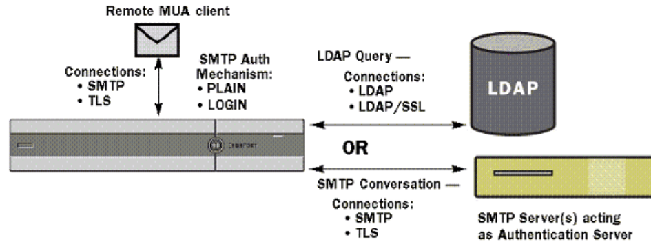
図 26-9 SMTP Auth のサポート:LDAP ディレクトリストアまたは SMTP サーバ
