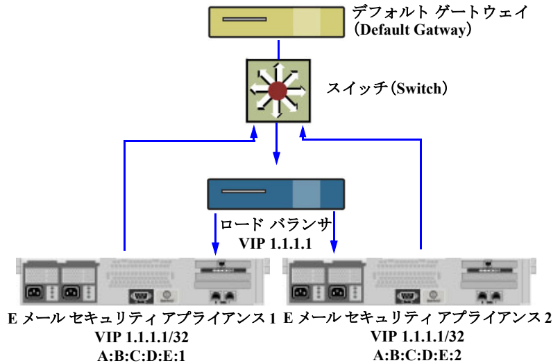
図 38-2 DSR を使用したスイッチ上の複数の E メール セキュリティ アプライアンス間でのロード バランス
