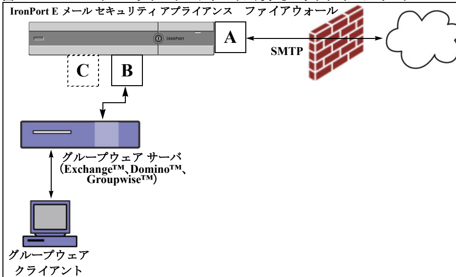
図 41-1 エンタープライズ ゲートウェイに対するブラック ホール リスナー
