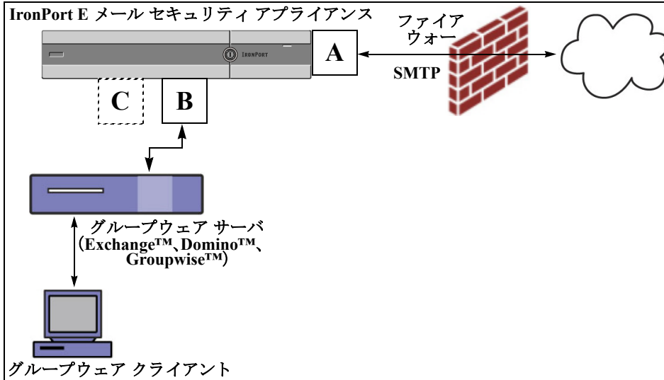
図 40-1 エンタープライズ ゲートウェイに対するブラック ホール リスナー
