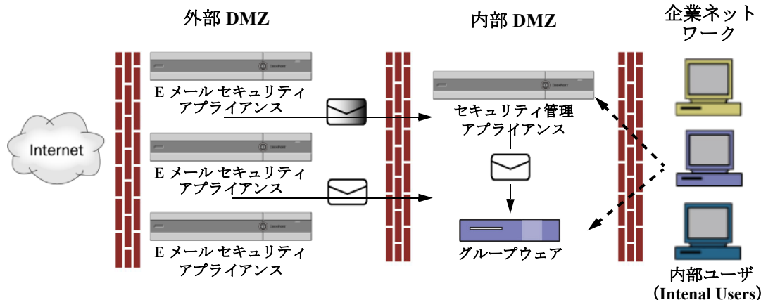
図 42-1 Cisco コンテンツ セキュリティ管理仮想アプライアンスによる一般的なネットワーク設定
