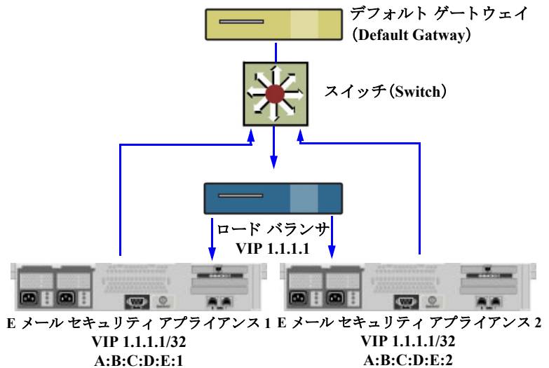
図 37-2 DSR を使用したスイッチ上の複数の E メール セキュリティ アプライアンス間でのロード バランス
