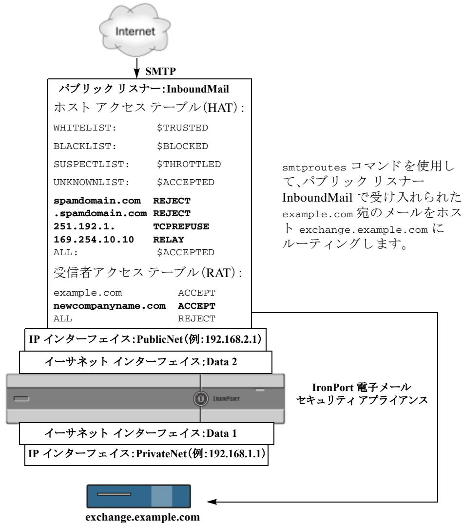
図 24-1 パブリック リスナー用に定義された SMTP ルート
