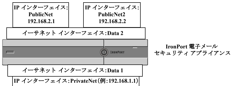
図 24-10 別のパブリック インターフェイスの追加
