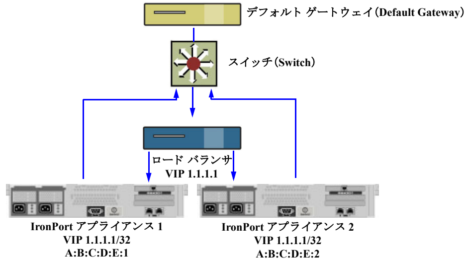
図 37-4 DSR を使用したスイッチ上の複数の E メール セキュリティ アプライアンス間でのロード バランス
