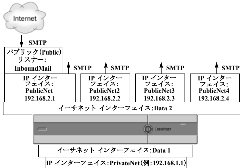
図 24-11 1つのイーサネット インターフェイス上にある4つの Virtual Gateway アドレス
