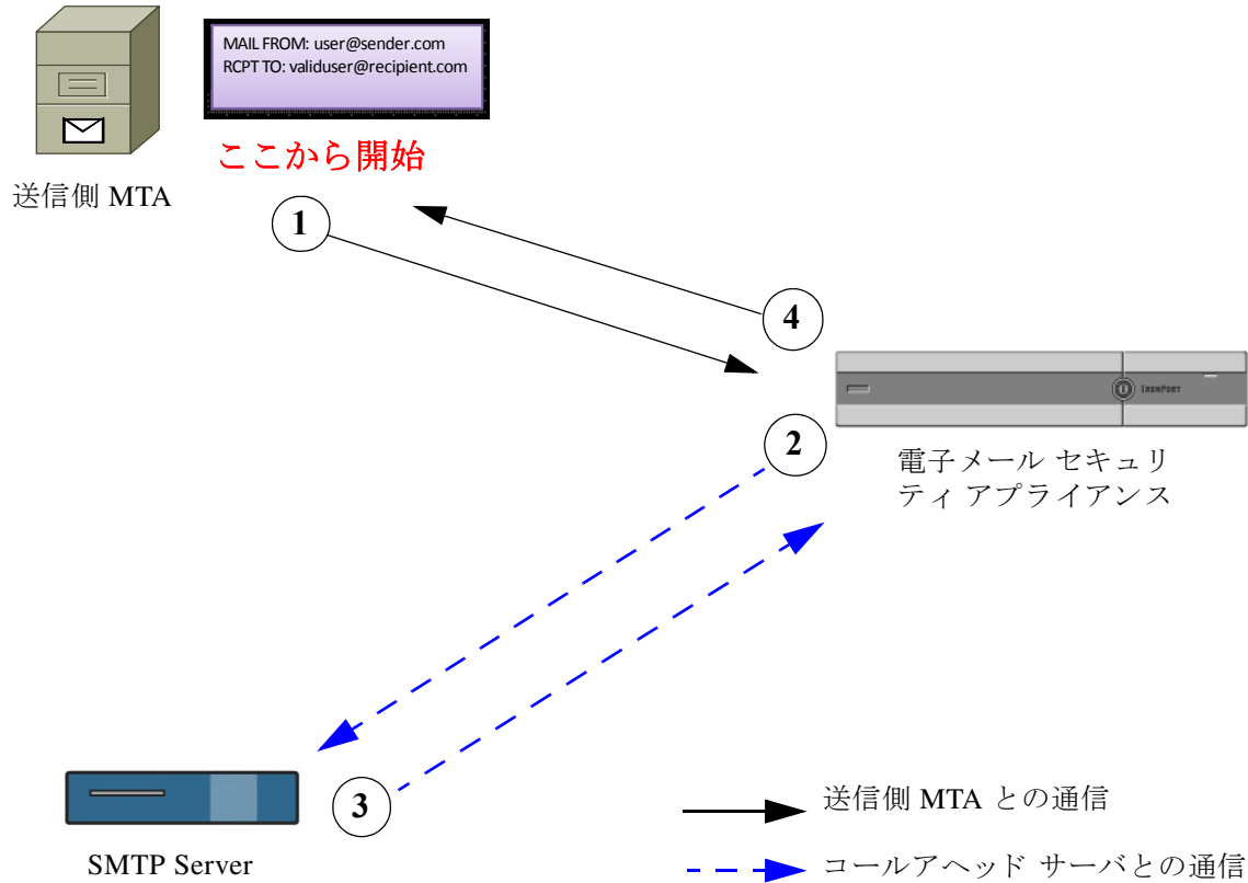
図 22-1 SMTP コールアヘッド サーバ通信のワークフロー
