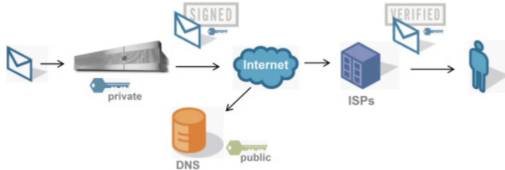
図 20-1 認証ワークフロー
