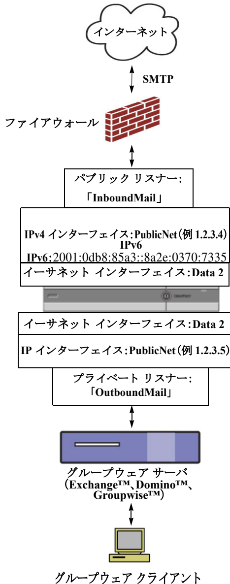
図 3-1 ファイアウォールの内側のシナリオ: リスナー 2 個の設定
