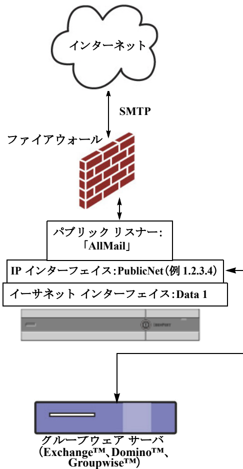
図 3-2 リスナー 1 個の設定
