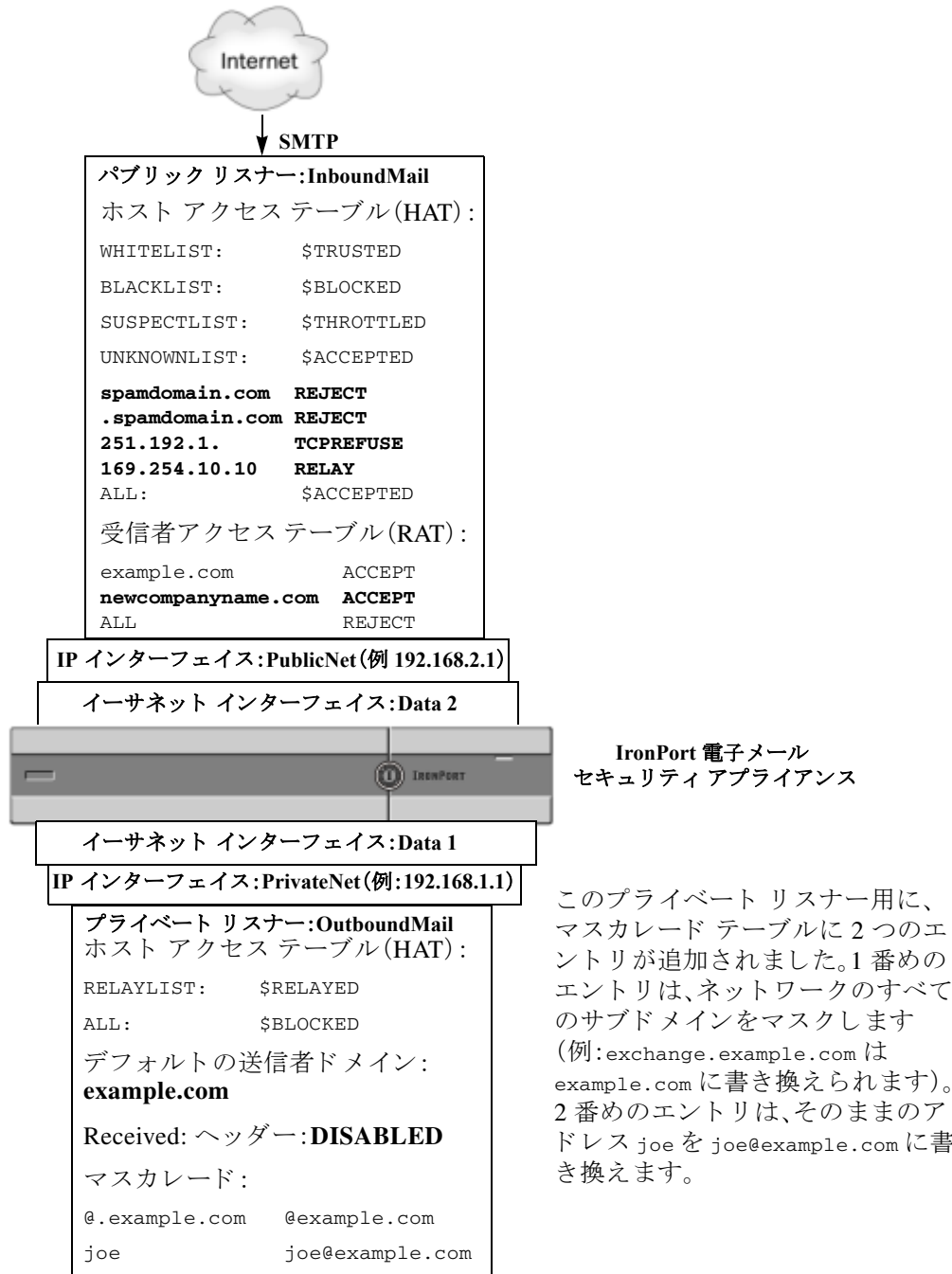
図 24-3 プライベート リスナー用に定義されたマスカレード
