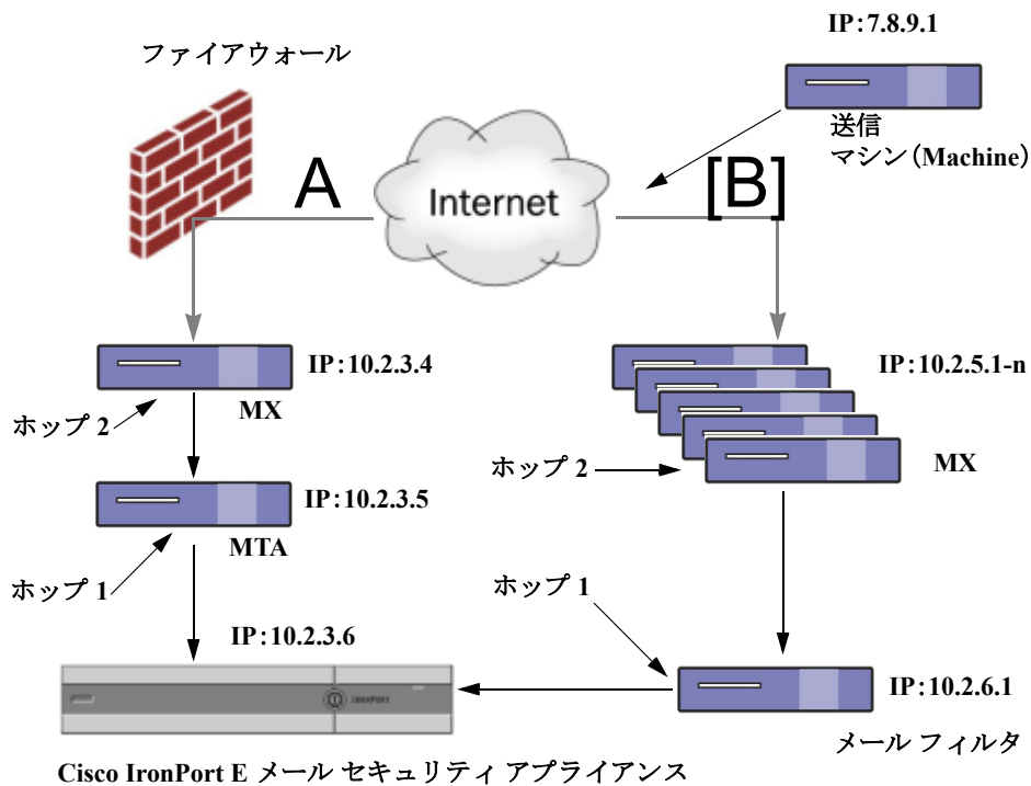
図 13-5 MX/MTA によるメール リレー:拡張
