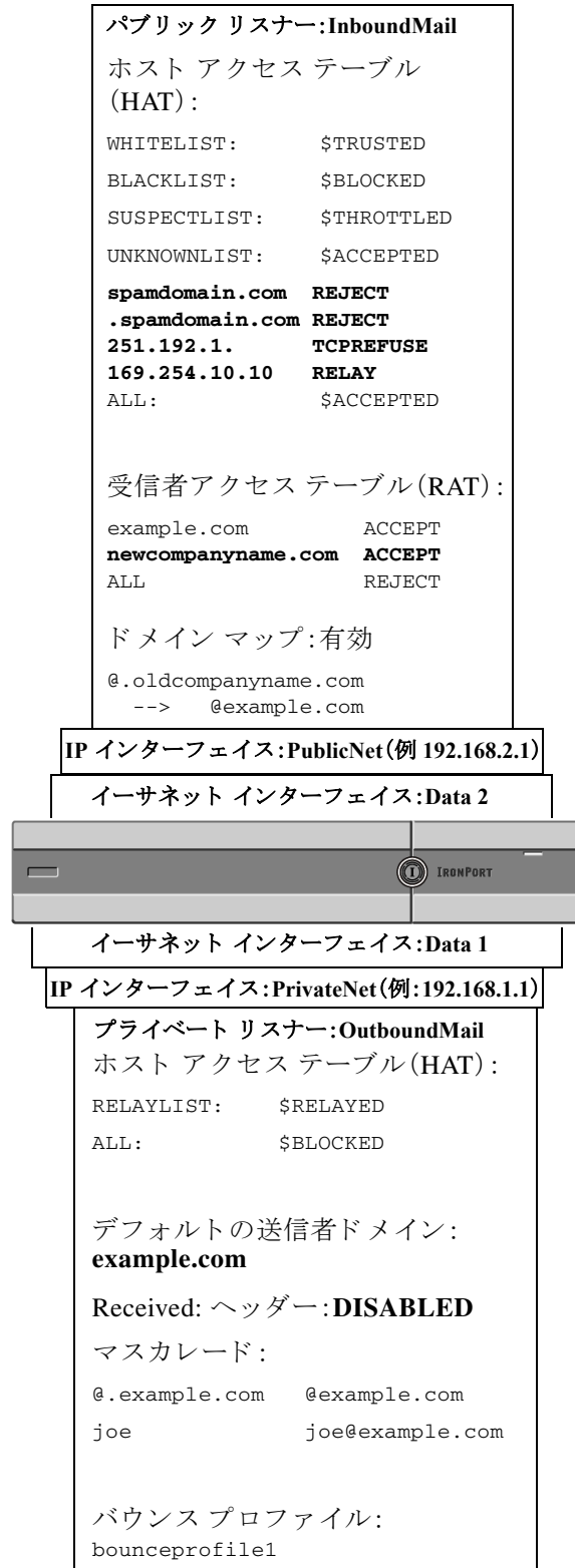
図 24-8 宛先および配信パラメータの設定
