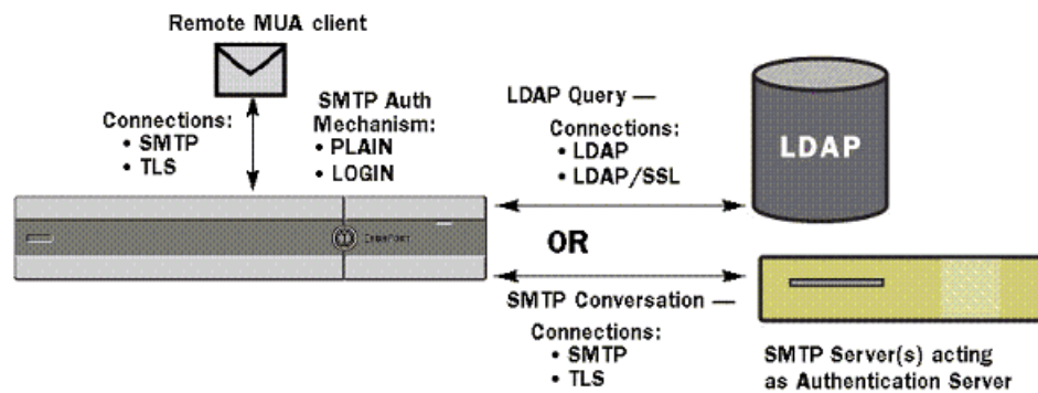
図 25-11 SMTP Auth のサポート:LDAP ディレクトリストアまたは SMTP サーバ
