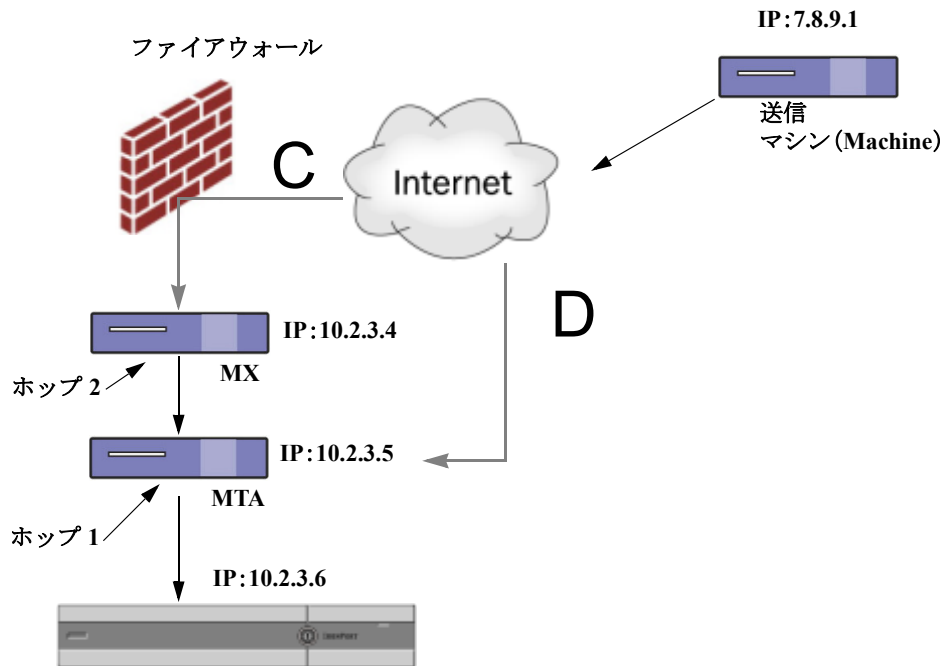
図13-6 MX/MTAによるメールリレー:不定ホップ数
