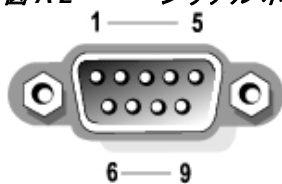
図 A-2 シリアルポートのピン番号
