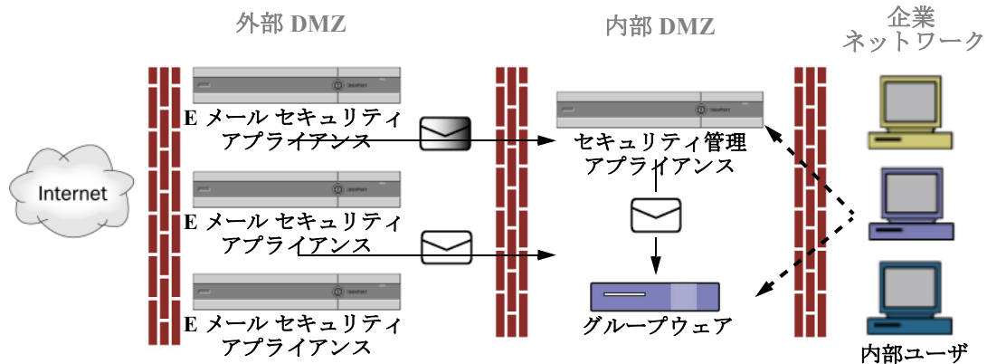
図 41-1 Cisco コンテンツ セキュリティ管理仮想アプライアンスによる一般的なネットワーク設定
