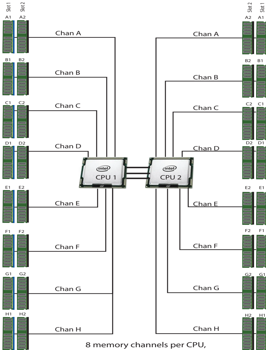
図 4 Cisco UCS X210c M7 コンピューティングノードのメモリ構成
