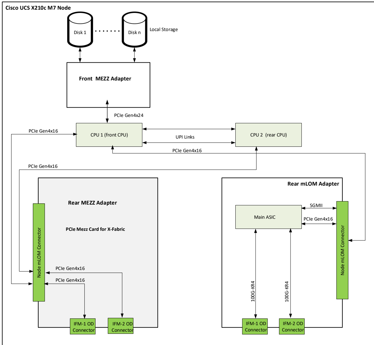
図 9 Cisco UCS X210c M7 コンピューティングノードの簡易ブロック図 (ドライブを装備した VIC 100G)
