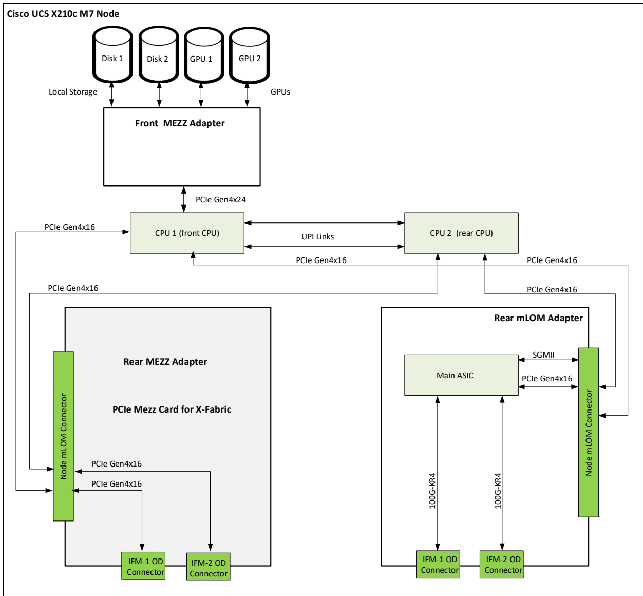
図 11 Cisco UCS X210c M7 コンピューティングノードの簡易ブロック図 (ドライブと GPU を装備した VIC 100G)
