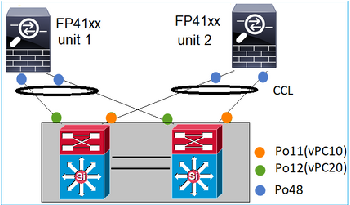
الاجلة 3. Port-Channel Terminated على FXOS
